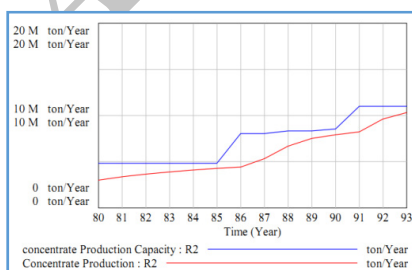
شکل ۱۸. ظرفیت و مقدار تولید کنسانتره
