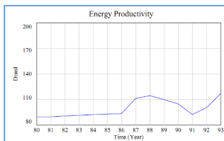
شکل ۲۲. بهره‌وری انرژی
