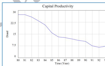
شکل ۲۱. بهره‌وری سرمایه
