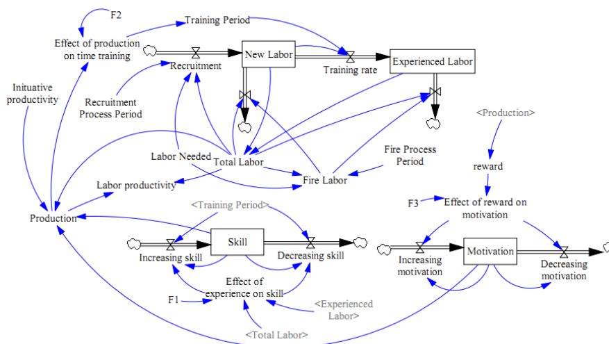
شکل ۹. مدل ریاضی بهره‌وری نیروی کار در معادن
