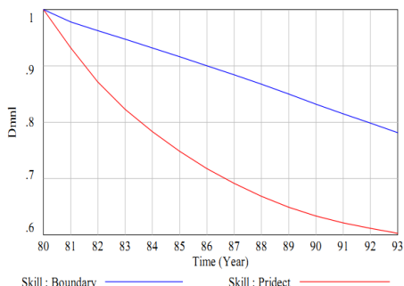
شکل ۱۶. آزمون شرایط حدی بهره‌وری اولیه
