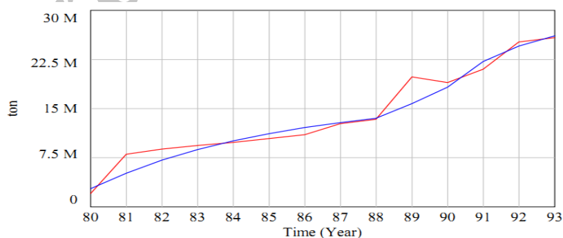
شکل ۱۴. اعتبارسنجی مدل به روش بازسازی رفتار مرجع
