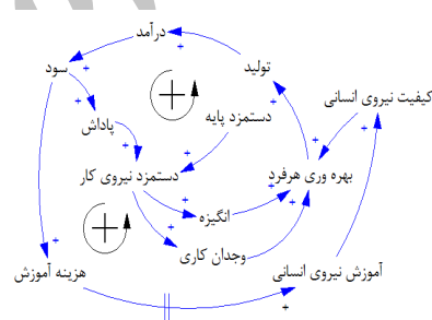
شکل ۶. حلقه‌های تقویت‌کننده R۳ و R۴
