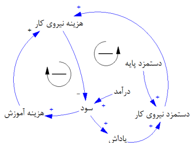
شکل ۷. حلقه‌های تعادلی B۲ و B۳
