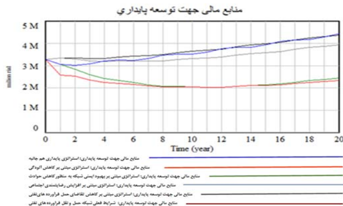
شکل ۱۸. نمودار مقایسه رفتار متغیر منابع مالی برای توسعه پایداری شرکت تحت استراتژی‌های مختلف
