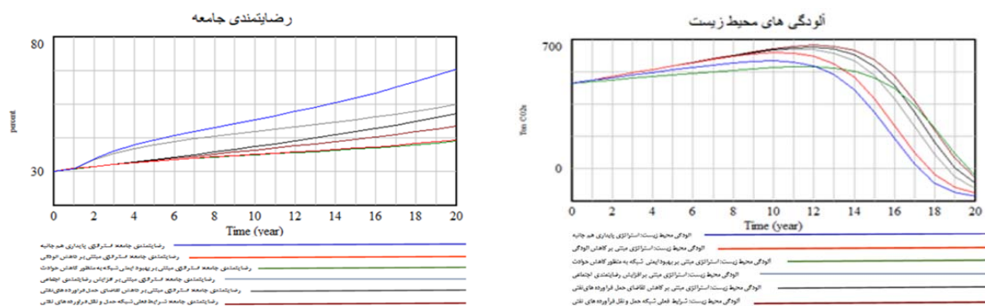
شکل ۱۷. نمودارهای مقایسه رفتار متغیر آلودگی محیط زیست و رضایتمندی جامعه تحت استراتژی‌های مختلف
