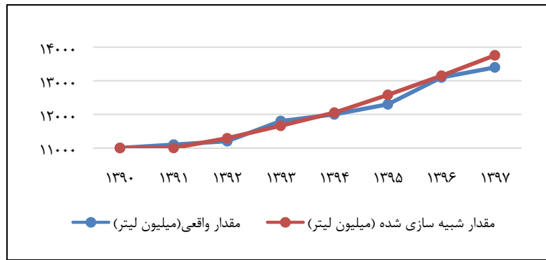
شکل ۱۵. مقادیر شبیه‌سازی و مرجع تأسیسات ذخیره‌سازی فراورده‌های نفتی
