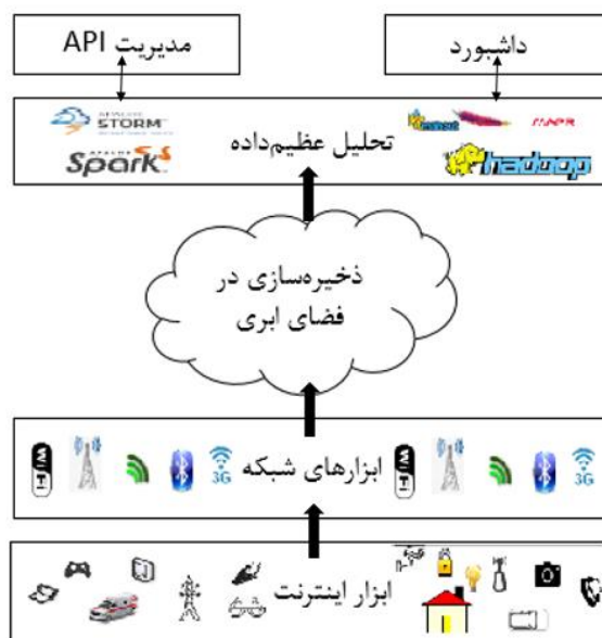
شکل ۱. معماری اینترنت اشیا برای تحلیل عظیم داده
