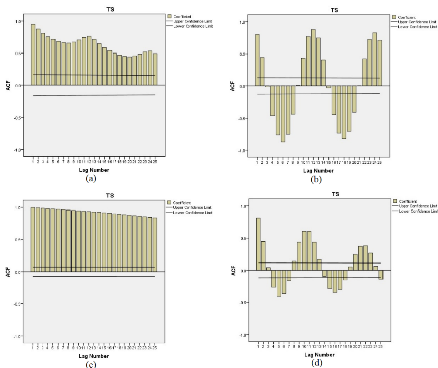
شکل ۲. نمودار خودهمبستگی چهار دسته سری زمانی (a) فصلی روندی؛ (b) فصلی؛ (c) روندی و (d) غیرخطی
