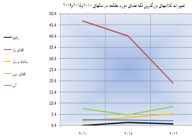
شکل ۷. تغییرات بزرگ‌ترین لکه در هر کلاس (منبع: نگارنده)
