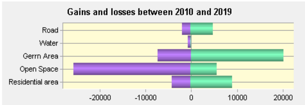
شکل ۱۴. تغییرات پوشش اراضی ۲۰۱۰-۲۰۱۹
