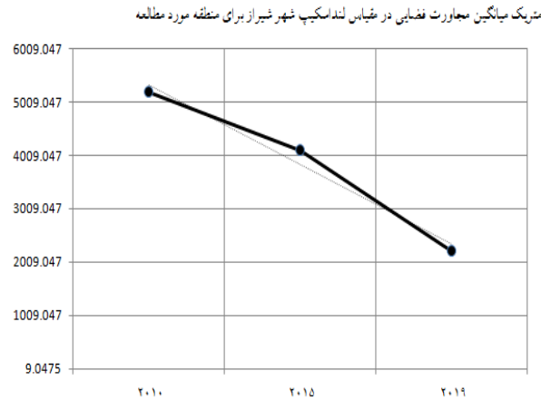
شکل ۱۰. تغییرات متریک مجاورت (منبع: نگارنده)
