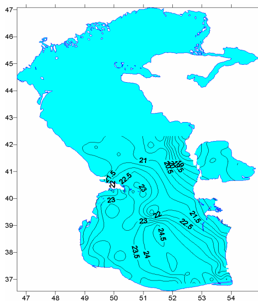
شکل ۴ خطوط هم دمای خزر جنوبی مربوط به روز ۲۰۰۳/۹/۲۹
