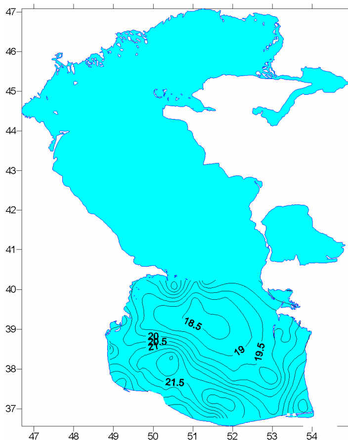
شکل ۲ خطوط هم دمای خزر جنوبی مربوط به روز ۲۰۰۵/۵/۲۴
