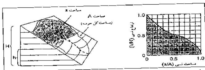
شکل ۱۶ شماتیک از یک حوضه آبریز فرضی و منحنی فرازنامی مربوط به آن. در شکل سمت چپ، پارامترهای لازم برای ترسیم منحنی فرازنامی نشان داده شده است.
