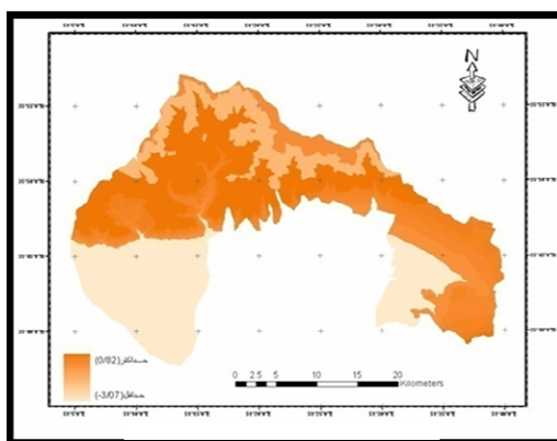
شکل ۱۳. وزن طبقات ارتفاعی در پیوند با حرکت‌های لغزشی
