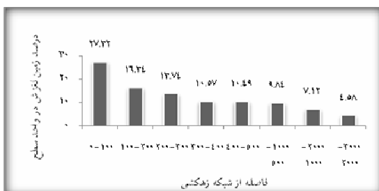
شکل ۱۱. هیستوگرام تراکم زمین لغزش‌ها در طبقات فاصله از شبکه زهکشی
