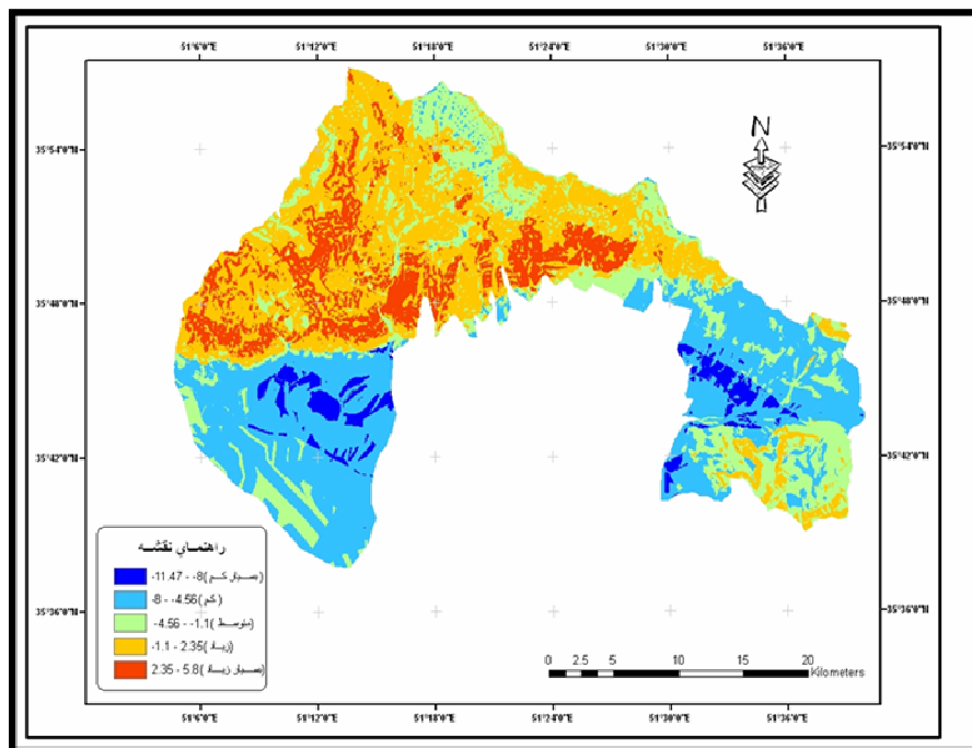
شکل ۲۰. نقشه نهایی پهنه‌بندی خطر زمین‌لغزش
