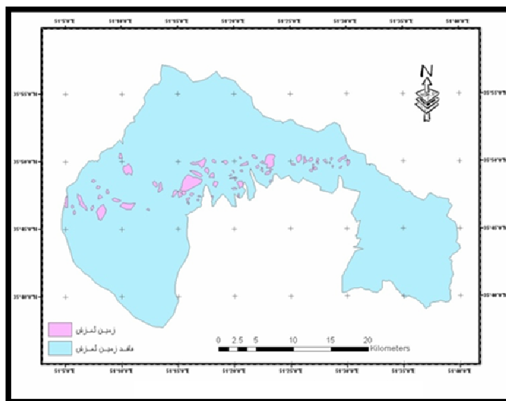
شکل ۳. زمین لغزش های برداشت شده در حوضه های کوهستانی
