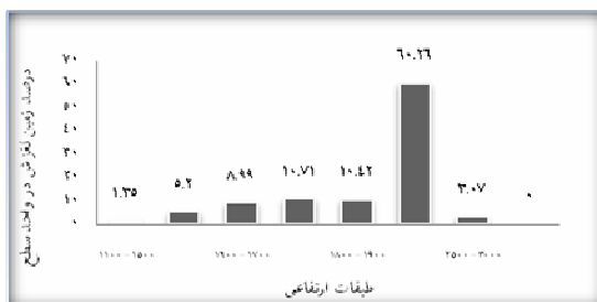
شکل ۵. هیستوگرام تراکم زمین لغزش ها در طبقات ارتفاعی
