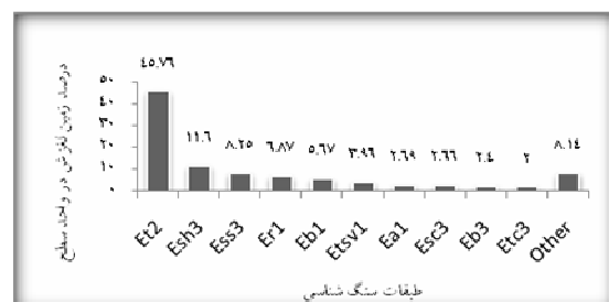
شکل ۴. هیستوگرام تراکم زمین لغزش ها در طبقات سنگ شناسی
