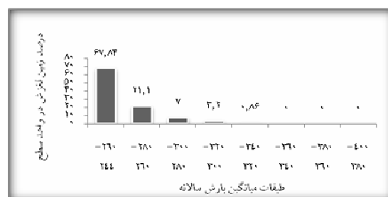
شکل ۸. هیستوگرام تراکم زمین لغزش‌ها در طبقات میانگین بارش سالانه
