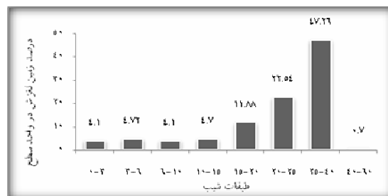
شکل ۶. هیستوگرام تراکم زمین لغزش‌ها در طبقات شیب
