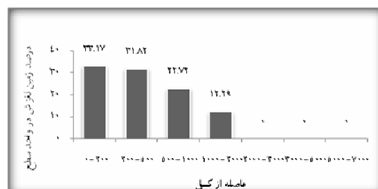
شکل ۱۰. هیستوگرام تراکم زمین لغزش‌ها در طبقات فاصله از کسب
