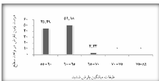
شکل ۹. هیستوگرام تراکم زمین لغزش‌ها در طبقات میانگین بارش شدید
