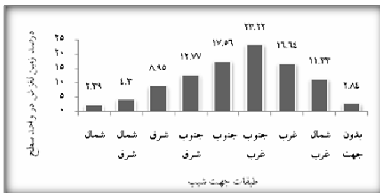
شکل ۷. هیستوگرام تراکم زمین لغزش‌ها در طبقات جهت شیب
