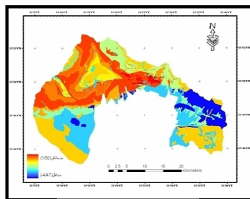
شکل ۱۲. وزن طبقات سنگ‌شناسی در پیوند با حرکت‌های لغزشی
