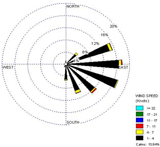
ج) گلباد سالانه ایستگاه اقدسیه
