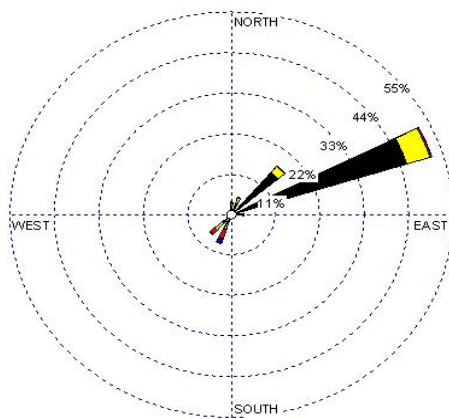
ب) گلباد سالانه ایستگاه فاطمی
