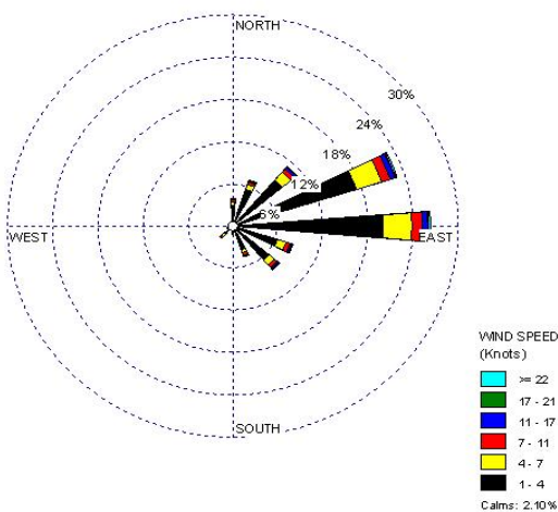
د) گلباد سالانه ایستگاه بازار
