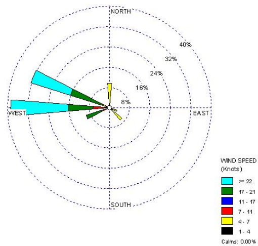
الف) گلباد سالانه ایستگاه مهرآباد
