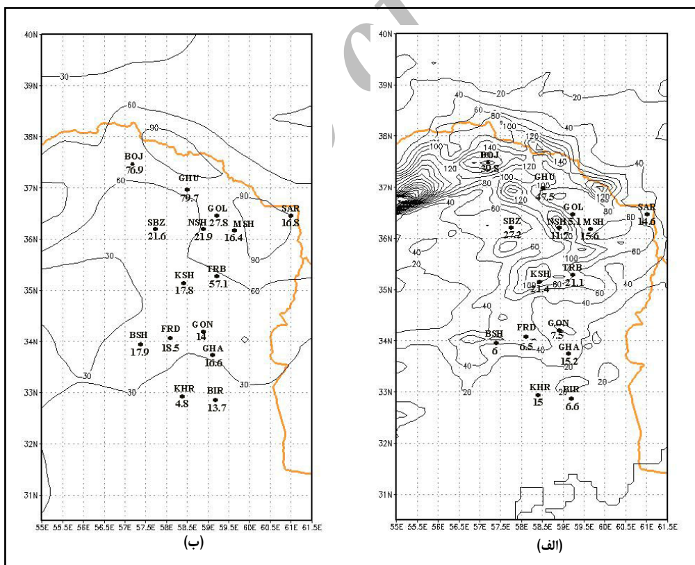
شکل ۲. مقایسه بارش مدل شده به وسیله مدل RegCM3 (خطوط ممتد) با بارش‌های واقعی (مقادیر پلات شده در زیر هر ایستگاه) الف) بدترین پاسخ مدل مربوط به پاییز ۱۹۹۳ با طرح‌واره گرل AS. ب) بهترین پاسخ مدل شده مربوط به پاییز ۱۹۹۹ با طرح‌واره کو. نام ایستگاه‌ها به اختصار با کد سه حرفی نشان داده شده است (مشهد: MSH، نیشابور: NSH، سبزوار: SBZ، بجنورد: BOJ، بیرجند BIR و ...)
