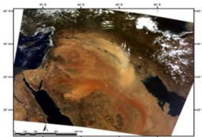
شکل ۱۷. الف) تصویر ماهواره‌ای روز ۲ ژوئن ۲۰۱۱ (برگرفته از سنجنده‌ی مادیس)
