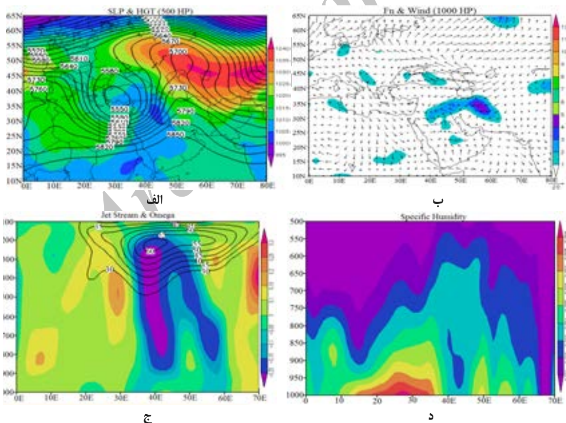
شکل ۶: الف) ارتفاع ژئوپتانسیل در تراز ۵۰۰ هکتوپاسکال (منحنی‌های ممتد)، فشار سطح دریا (سطوح رنگی) در ۳ آوریل ۲۰۱۱. ب) تابع جبهه‌زایی بر حسب 10^{-4} K \cdot m^{-1} \cdot S^{-1} و بردار باد در تراز ۱۰۰۰ هکتوپاسکال در ۳ آوریل. ج) امگا به پاسکال بر ثانیه (سطوح رنگی) و موقعیت جت‌باد (منحنی‌های هم سرعت به متر بر ثانیه)، در عرض ۳۵ درجه در ساعت ۰۰ زولو، ۴ آوریل ۲۰۱۱. د) نمایه‌ی قائم رطوبت ویژه به گرم در کیلوگرم (سطوح رنگی).
