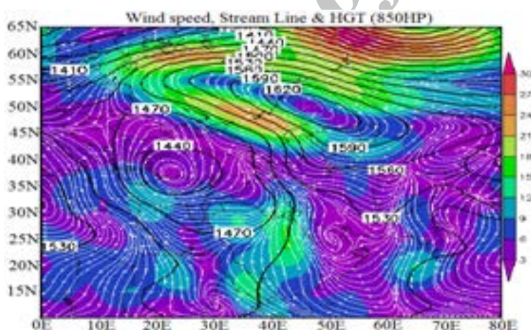
شکل ۷. ارتفاع ژئوپتانسیل (منحنی‌های ممتد)، سرعت باد به متر بر ثانیه (سطوح رنگی) و خطوط جریان هوا در تراز ۸۵۰ هکتوپاسکال در ساعت ۰۰ زولو در ۴ آوریل ۲۰۱۱
