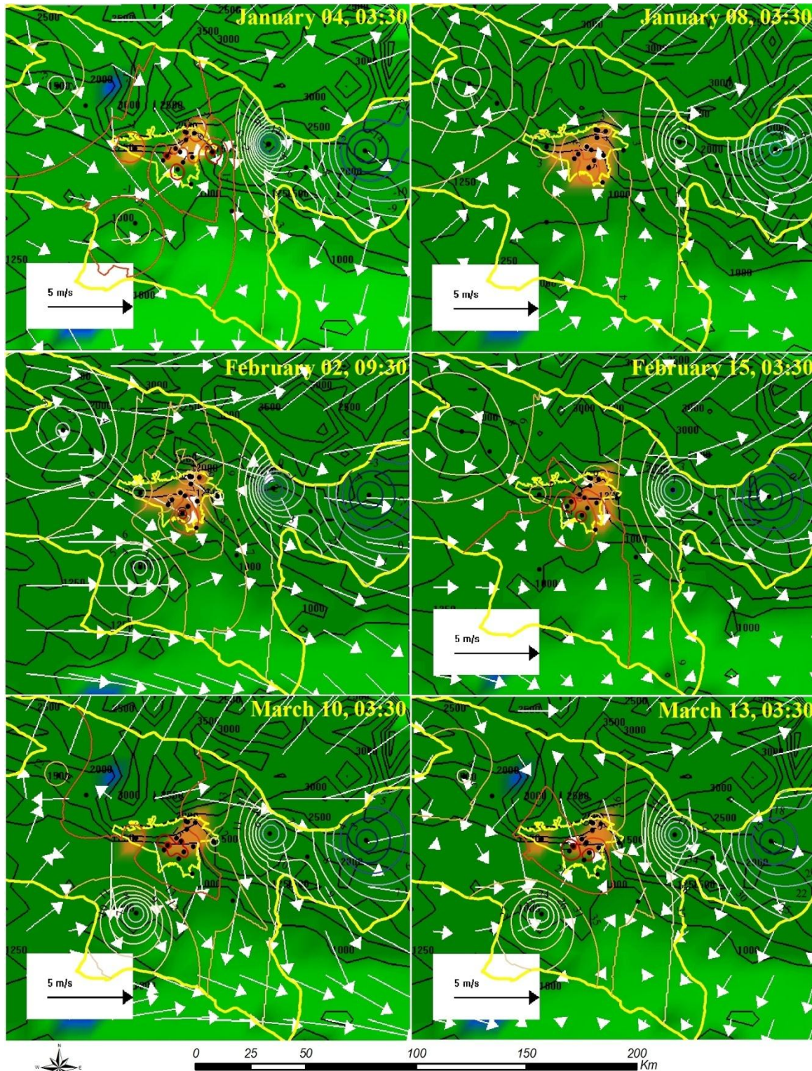
شکل ۳. گستره‌ی مکانی جزیره گرمایی شهری در پیشینه‌ی شدت آن در فصل زمستان
