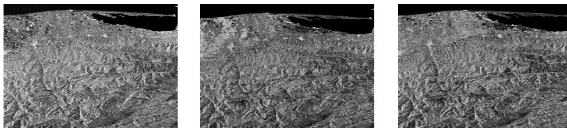
شکل ۳. تصاویر رادارست از منطقه مورد بررسی: الف) تاریخ ۱۹۹۸/۵/۵؛ ب) تاریخ ۱۹۹۸/۶/۲۲؛ ج) تاریخ ۱۹۹۸/۸/۲۶
