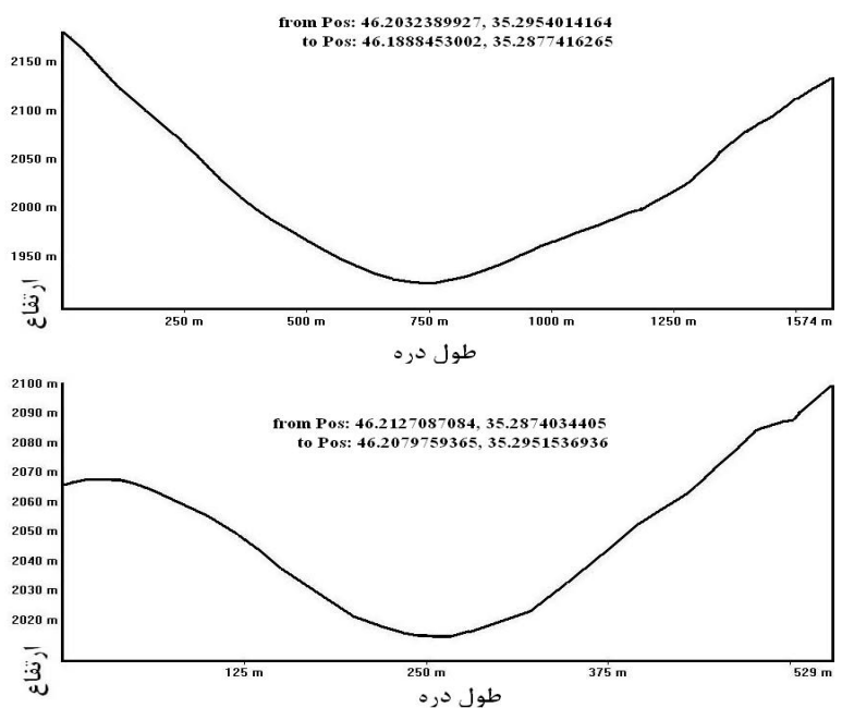
شکل ۸. نیم‌رخ عرضی نمونه دره‌های محدوده زروه که U شکل هستند
