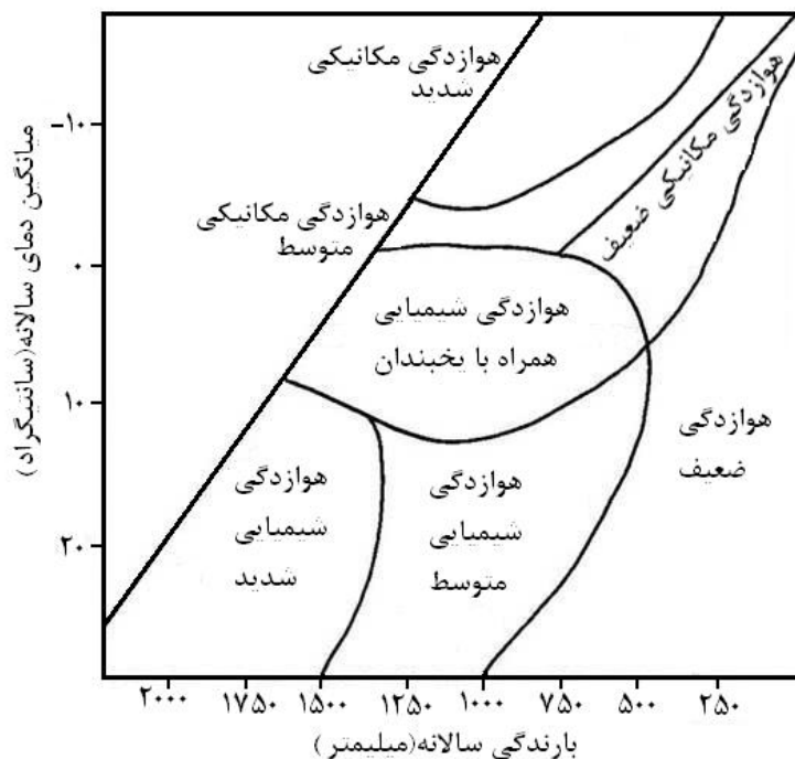
شکل ۲. رژیم‌های هوازدگی پلتیر
