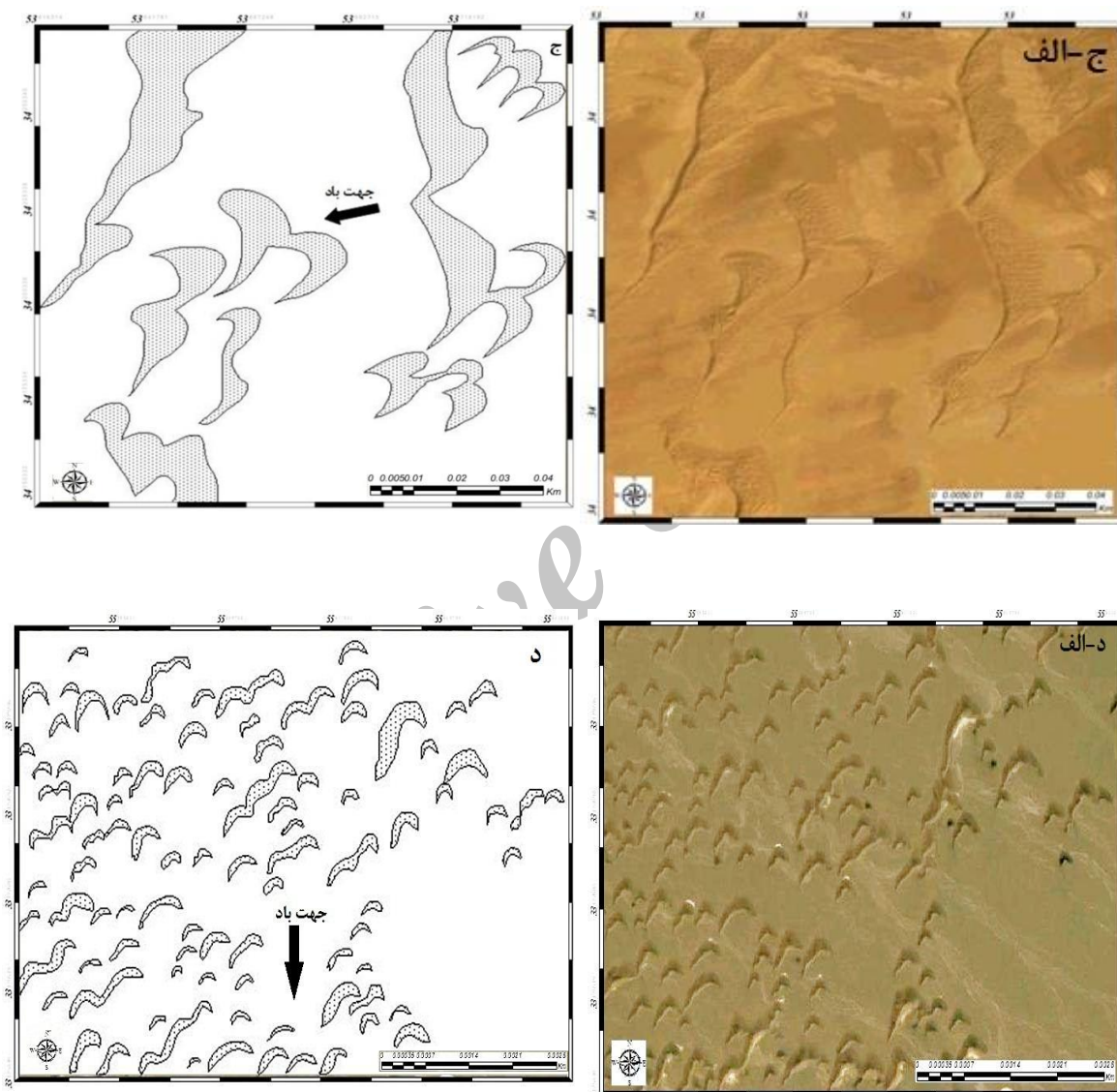
شکل ۶. اثر بادها در ایجاد مورفولوژی ماسه‌ای شمال ریگ جن (ج) و غرب ریگ سرگردان (د)، سال ۲۰۱۱
