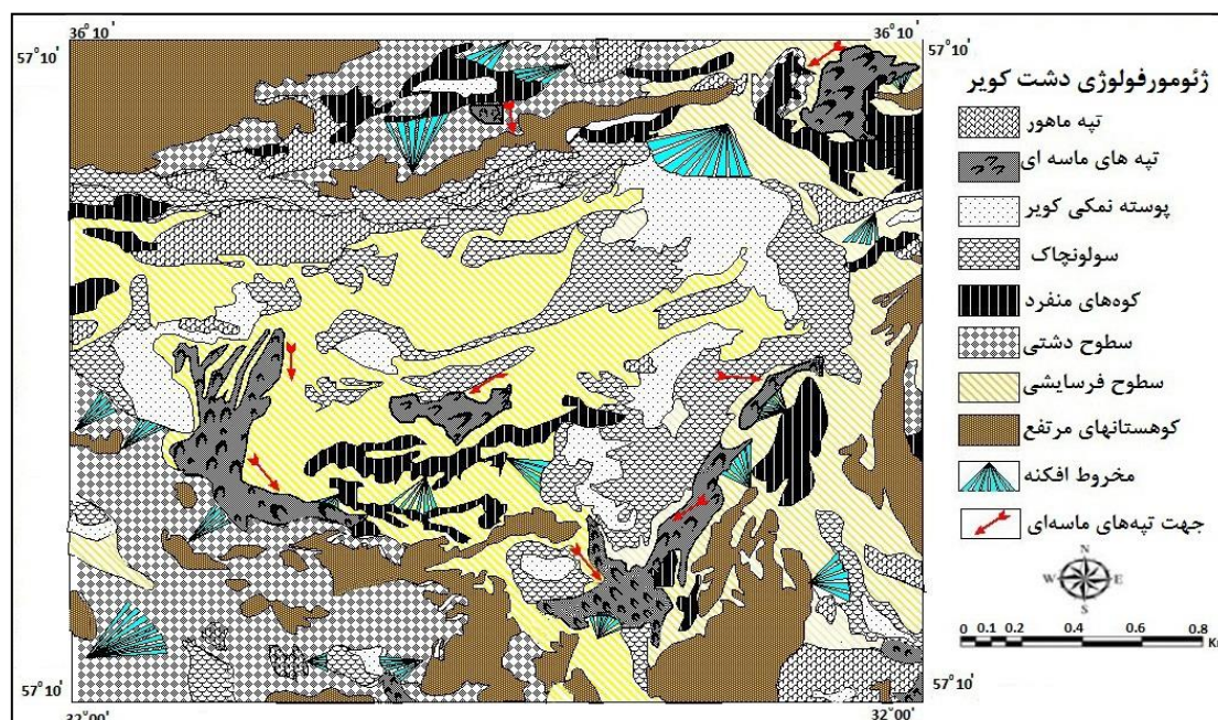
شکل ۳. نقشه ژئومورفولوژی پهنه دشت کویر (نقشه ۱:۲۵۰۰۰۰۰ ژئومورفولوژی ایران)
