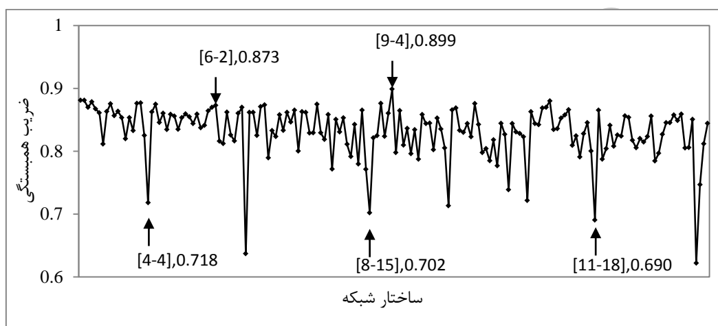
شکل ۲. ضریب همبستگی ترکیب‌های مختلف نرون‌های ورودی و مخفی برای سری زمانی SPI12 بندرانزلی بر اساس مدل DMSNN (ساختار شبکه: [a-b]، تعداد نرون ورودی: a = ۱ تا ۱۲، تعداد نرون لایه مخفی: b = ۱ تا ۲a+۱)
