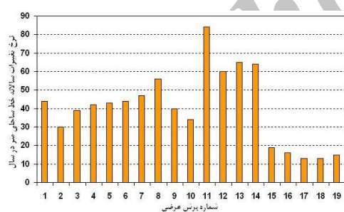
شکل ۵. نمودار ستونی مقدار تغییرات سالانه خط ساحلی به روش EPR در ۱۹ پرتو بررسی شده
