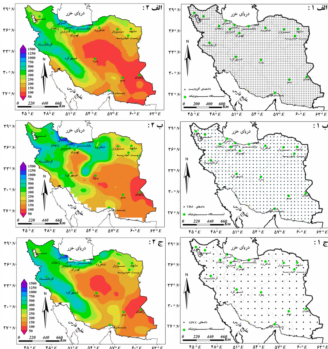
شکل ۵. میانگین بلندمدت بارش سالانه ایران براساس داده‌های آفرودیت (الف ۲، ۱۹۵۱-۲۰۰۷)، UDel (ب ۲، ۱۹۴۸-۲۰۱۰) و GPC (ج ۲، ۱۹۴۸-۲۰۱۳) و موقعیت مراکز هر شبکه در داده‌های آفرودیت (الف ۱)، UDel (ب ۱) و GPC (ج ۱)
