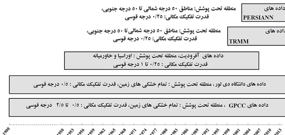
شکل ۱. طول دوره زمانی پرکاربردترین داده‌های بارش به همراه برخی ویژگی‌های آن‌ها
