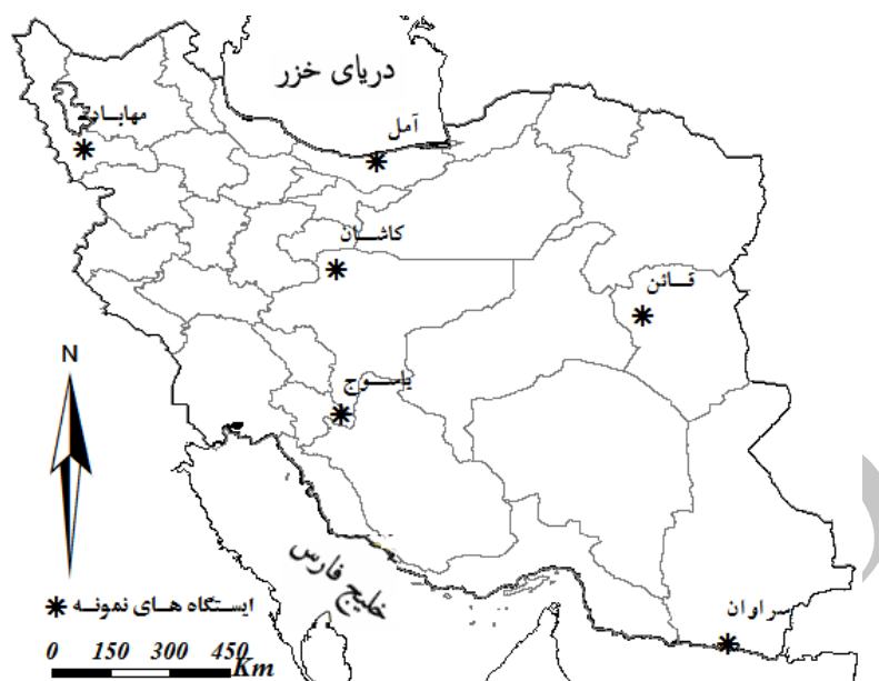
شکل ۹. موقعیت ایستگاه‌های نمونه به منظور ارزیابی داده‌های مورد نظر در رابطه با سری‌های زمانی کوتاه مدت
