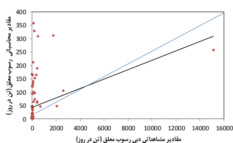
شکل ۸. مقادیر محاسباتی و مشاهداتی رسوب معلق به‌دست‌آمده از منحنی سنجه رسوب
