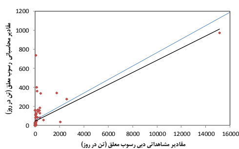
شکل ۱۰. مقادیر محاسباتی و مشاهداتی دبی رسوب معلق به‌دست‌آمده از روش فصلی
