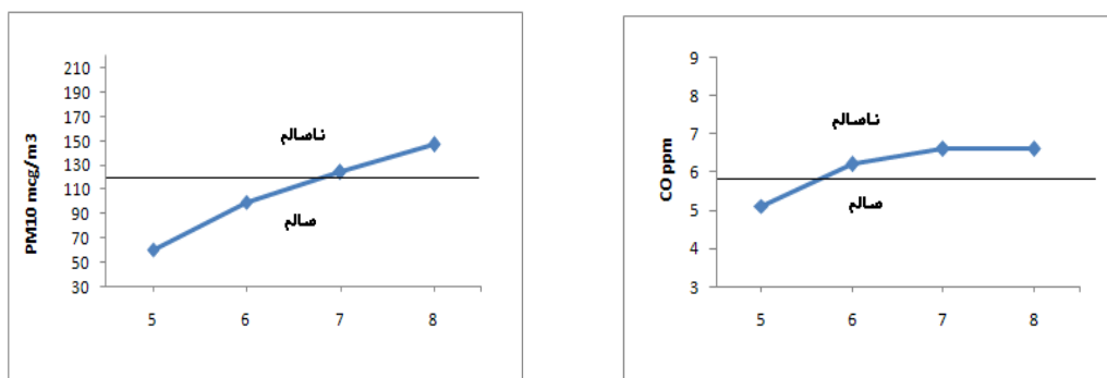
شکل ۱۴. نمودار غلظت PM 10 و CO در روزهای آلوده از پنجم تا هشتم دسامبر ۲۰۰۸
