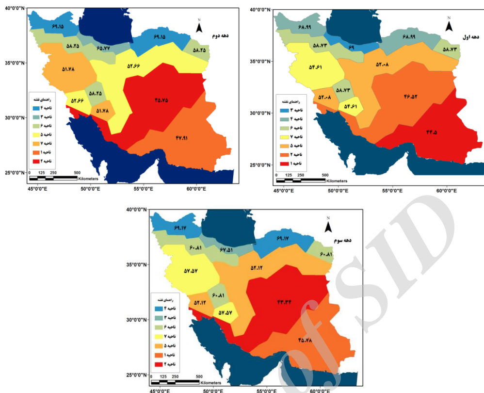
شکل ۷. تغییرات دهه‌ای نمایه یکنواختی بارش در ایران
