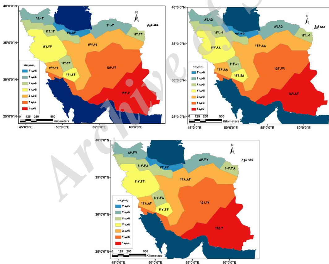
شکل ۵. تغییرات ضریب بارش ایران در دهه‌های مختلف
