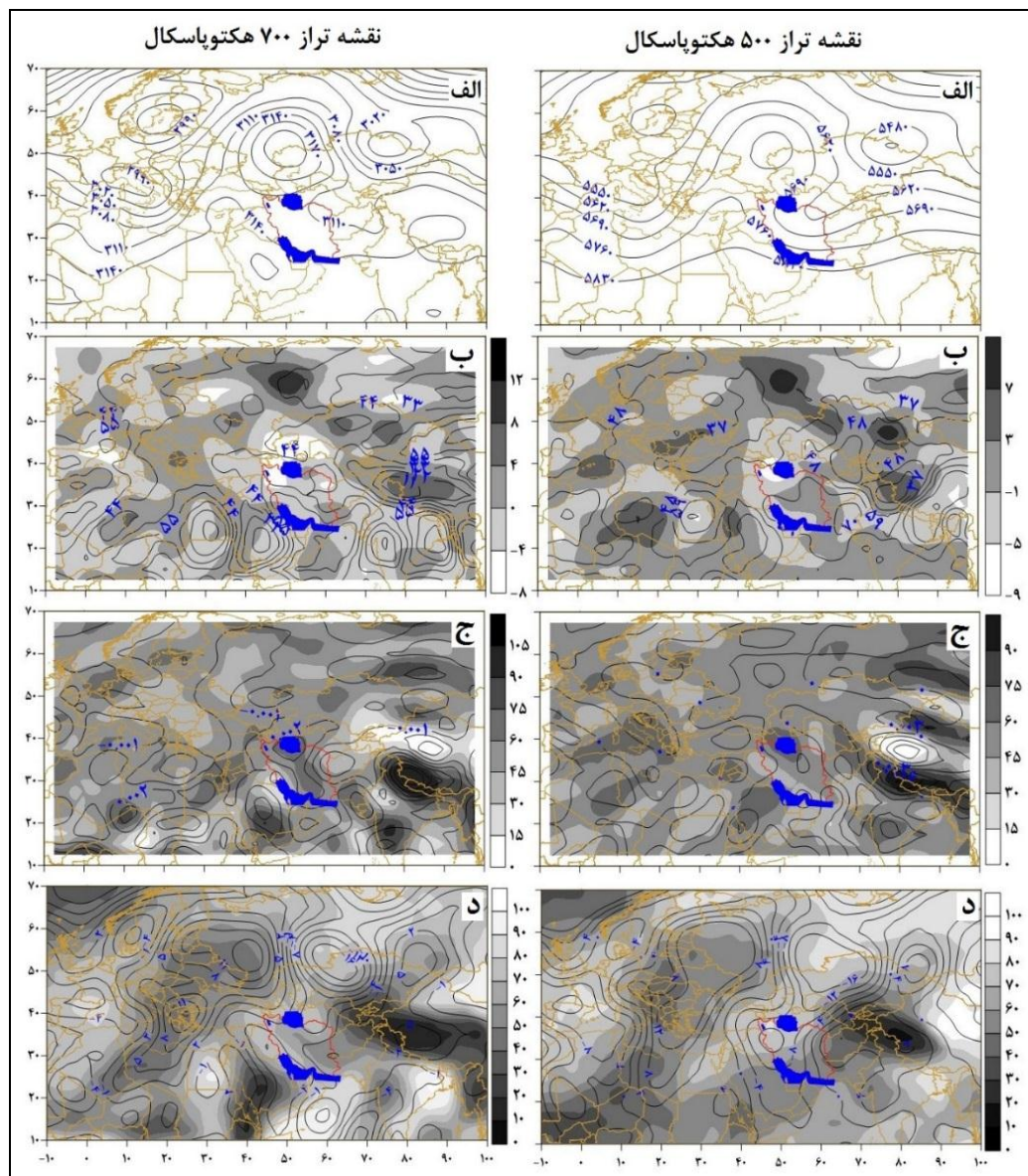
شکل ۱۰. توزیع ارتفاع تراز ۵۰۰ (الف) و ۷۰۰ (الف) هکتوپاسکال؛ فرافت دمایی (درجه سلسیوس) و فراوانی (درصد) آن در تراز ۵۰۰ (ب) و ۷۰۰ (ب) هکتوپاسکال؛ هم‌گرایی و واگرایی و فراوانی آن (درصد) در تراز ۵۰۰ (ج) و ۷۰۰ (ج) هکتوپاسکال؛ باد نصف‌النهاری (متر بر ثانیه) و فراوانی آن (درصد) در تراز ۵۰۰ (د) و ۷۰۰ (د) هکتوپاسکال برای روز نماینده چهارم ۱۳۶۶/۹/۸
