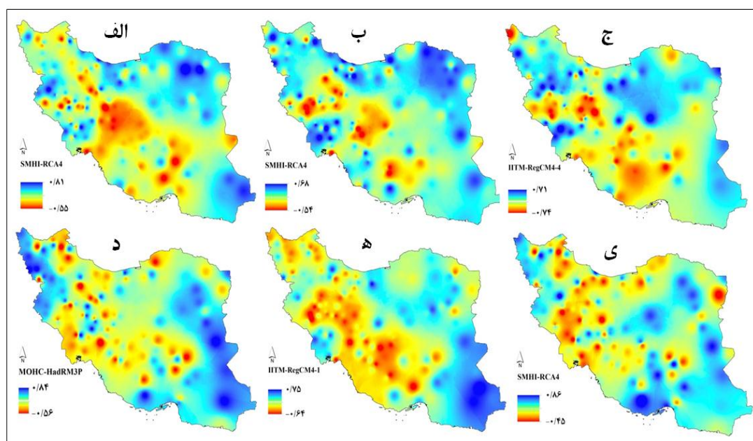
شکل ۸. همبستگی داده‌های واقعی بارش با خروجی مدل‌های منطقه‌ای آب و هوا در پهنه ایران: (الف) MNA-0.22؛ (ب) MNA-0.44؛ (ج) WAS-0.44
