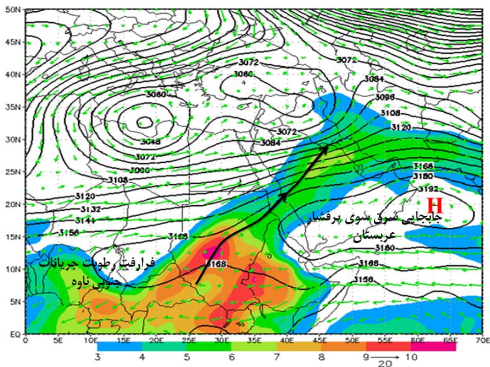
شکل ۱۰. نقشه ارتفاع ژئوپتانسیل (m)، نم و یژه (g/kg)، و نقشه جریان (m/s) تراز ۷۰۰ هکتوپاسکال روز ۱۲ مارس ۱۹۹۷
