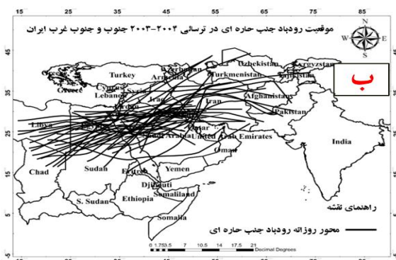
شکل ۴. موقعیت رودباد جنب‌حاره‌ای در ترسالی ۱۹۹۶-۱۹۹۷ (الف) و ۲۰۰۳-۲۰۰۴ (ب) در جنوب و جنوب‌غرب ایران تراز ۲۵۰ هکتوپاسکال استقرار رودباد جنب‌حاره‌ای در این منطقه جغرافیایی سبب می‌شود جنوب و جنوب‌غرب ایران در مناسب‌ترین موقعیت (شمال‌غرب، سمت چپ خروجی) رودباد جنب‌حاره‌ای قرار بگیرد.
