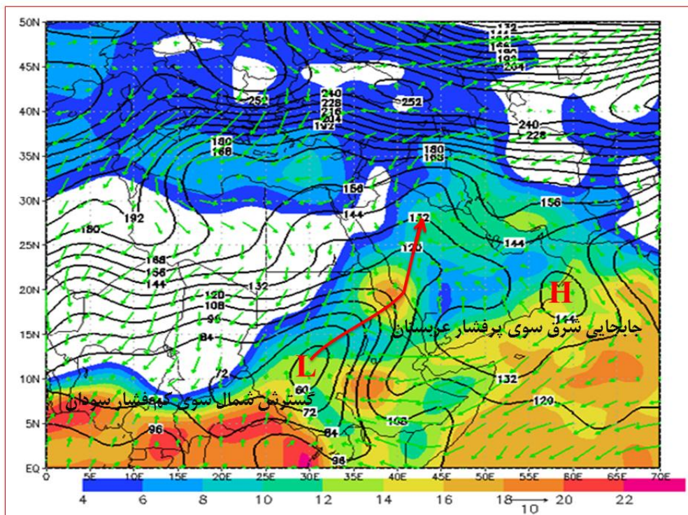
شکل ۸. نقشهٔ ارتفاع ژئوپتانسیل (m)، نم و بزه (g/kg)، و نقشهٔ جریان (m/s) تراز ۱۰۰۰ هکتوپاسکال روز ۱۲ مارس ۱۹۹۷
