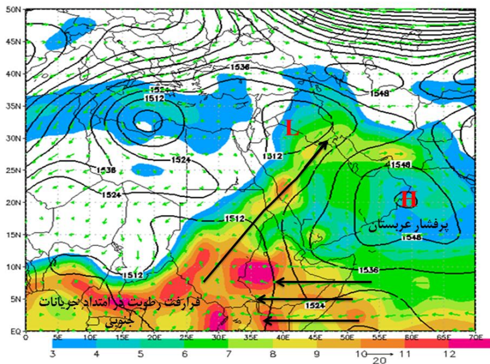
شکل ۹. نقشه ارتفاع ژئوپتانسیل (m)، نم و یژه (g/kg)، و نقشه جریان (m/s) تراز ۸۵۰ هکتوپاسکال روز ۱۲ مارس ۱۹۹۷
