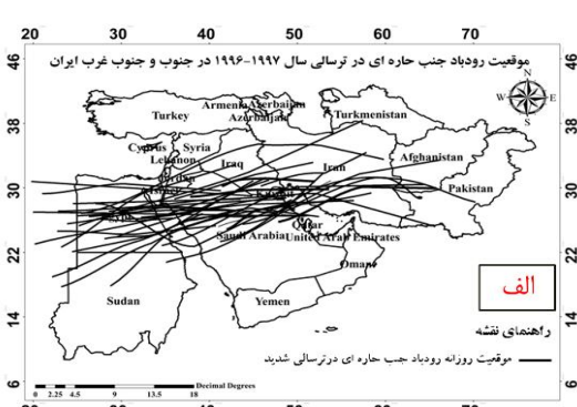
شکل ۴. موقعیت رودباد جنب‌حاره‌ای در ترسالی ۱۹۹۶-۱۹۹۷ (الف) و ۲۰۰۳-۲۰۰۴ (ب) در جنوب و جنوب‌غرب ایران تراز ۲۵۰ هکتوپاسکال استقرار رودباد جنب‌حاره‌ای در این منطقه جغرافیایی سبب می‌شود جنوب و جنوب‌غرب ایران در مناسب‌ترین موقعیت (شمال‌غرب، سمت چپ خروجی) رودباد جنب‌حاره‌ای قرار بگیرد.
