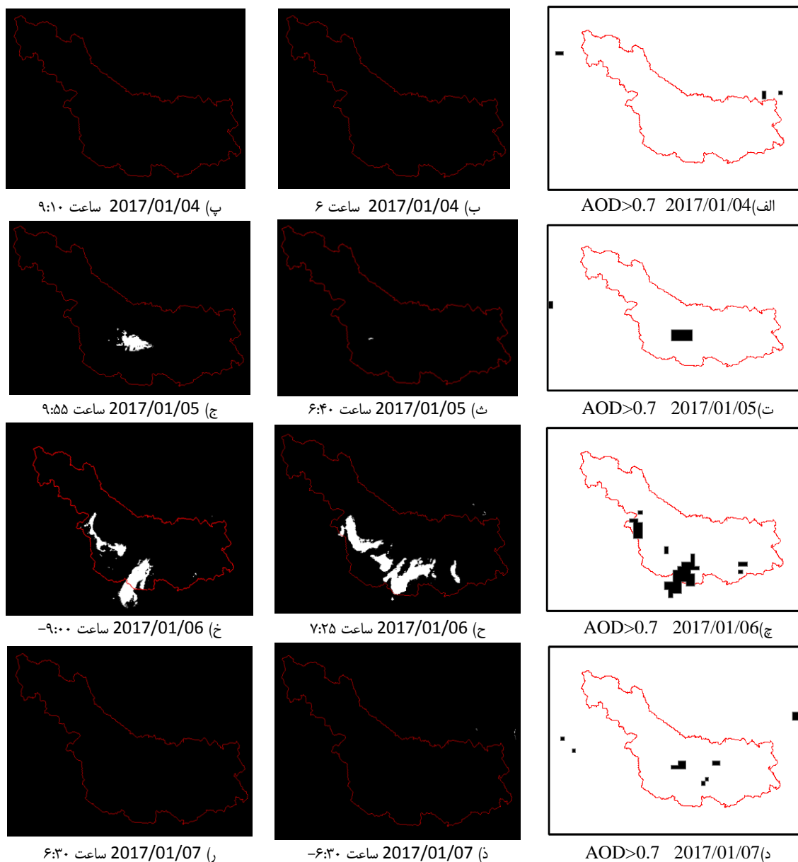
شکل ۶. مقایسه دقت روش زاو و همکاران (۲۰۱۰) و AOD در آشکارسازی گرد و غبار طی دوره ۲۰۱۷/۰۱/۰۴ تا ۲۰۱۷/۰۱/۰۸. تصاویر «الف»، «ب»، «ج»، «د»، «ه» و «ز» بخش های سیاه رنگ پیسل های بارزش AOD>0.7 و نشان دهنده تراکم گرد و غبار بیشتر هستند. سایر تصاویر نتیجه آشکارسازی گرد و غبار با رنگ سفید نشان داده شده است
