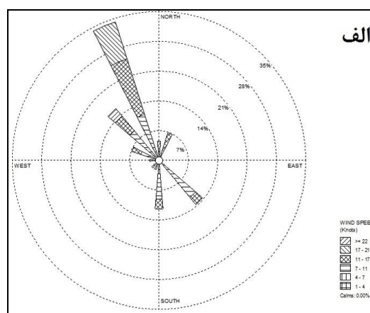
شکل ۳. گل‌باد و گل‌ماسه سالانه در ایستگاه سینوپتیک بافق (دوره آماری ۱۳۷۶-۱۳۹۶)
