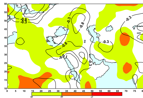
شکل ۳. همگرایی تراز ۱۰۰۰ هکتوپاسکال (بهنه‌های رنگی) و واگرایی تراز ۵۰۰ هکتوپاسکال (خطوط هم مقدار) بر حسب 10^{-10} \text{ s}^{-1} ساعت ۰۰۰۰ گرینویچ روز ۱۹۷۴/۱۲/۵
