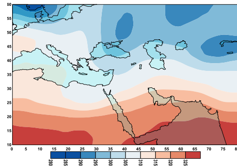
شکل ۱. الگوی دمای پتانسیل تراز ۵۰۰ هکتوپاسکال بر حسب کلونین در ساعت ۰۰۰۰ گرینویچ روز ۱۹۷۴/۱۲/۵
