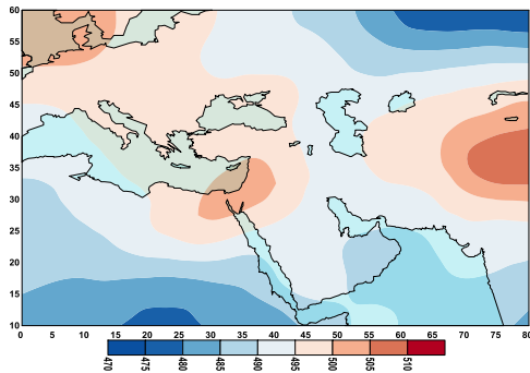
شکل ۲. الگوی دمای پتانسیل تراز ۵۰۰ هکتوپاسکال بر حسب کلونین در ساعت ۰۰۰۰ گرینویچ روز ۱۹۷۴/۱۲/۵
