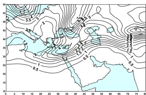
شکل ۱۰. توزیع مکانی تاوایی پتانسیلی راسبی- ارتل سطح هم‌انرژی ۳۳۰ کلون، در ساعت ۰۰۰۰ گرینویچ روز ۱۹۷۴/۱۲/۵
