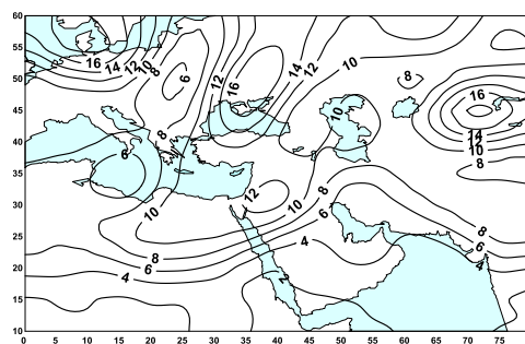
شکل ۷. توزیع مکانی تاوایی مطلق تراز ۵۰۰ هکتوپاسکال بر حسب 10^{-5} \text{ s}^{-1} در ساعت ۰۰۰۰ گرینویچ روز ۱۹۷۴/۱۲/۵
