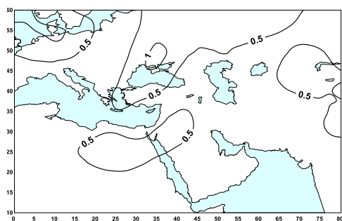
شکل ۸. توزیع مکانی تاوایی پتانسیلی راسبی- ارتل تراز ۵۰۰ هکتوپاسکال بر حسب 10^{-5} \text{ s}^{-1} در ساعت ۰۰۰۰ گرینویچ روز ۱۹۷۴/۱۲/۵
