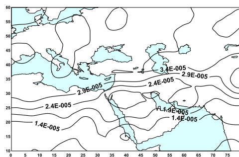
شکل ۹. توزیع مکانی تاوایی پتانسیلی راسبی- ارتل تراز ۵۰ هکتوپاسکال در ساعت ۰۰۰۰ گرینویچ روز ۱۹۷۴/۱۲/۵
