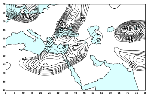
شکل ۶. توزیع مکانی تاوایی نسبی تراز ۵۰۰ هکتوپاسکال بر حسب 10^{-5} \text{ s}^{-1} ساعت ۰۰۰۰ گرینویچ روز ۱۹۷۴/۱۲/۵
