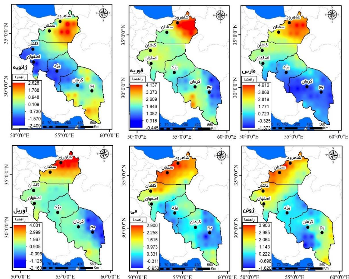
شکل ۵. روند تغییر سرعت باد در ایران مرکزی با استفاده از آزمون من-کندال براساس پایگاه ECMWF نسخه ERA-Interim
