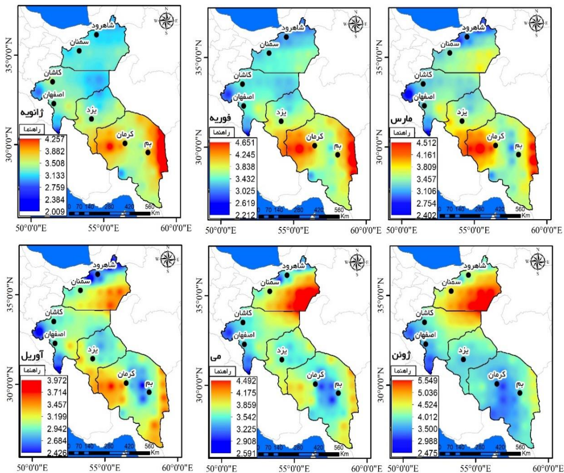
شکل ۳. پراکنش مکانی باد (m/s) در ایران مرکزی براساس پایگاه ECMWF نسخه ERA-Interim
