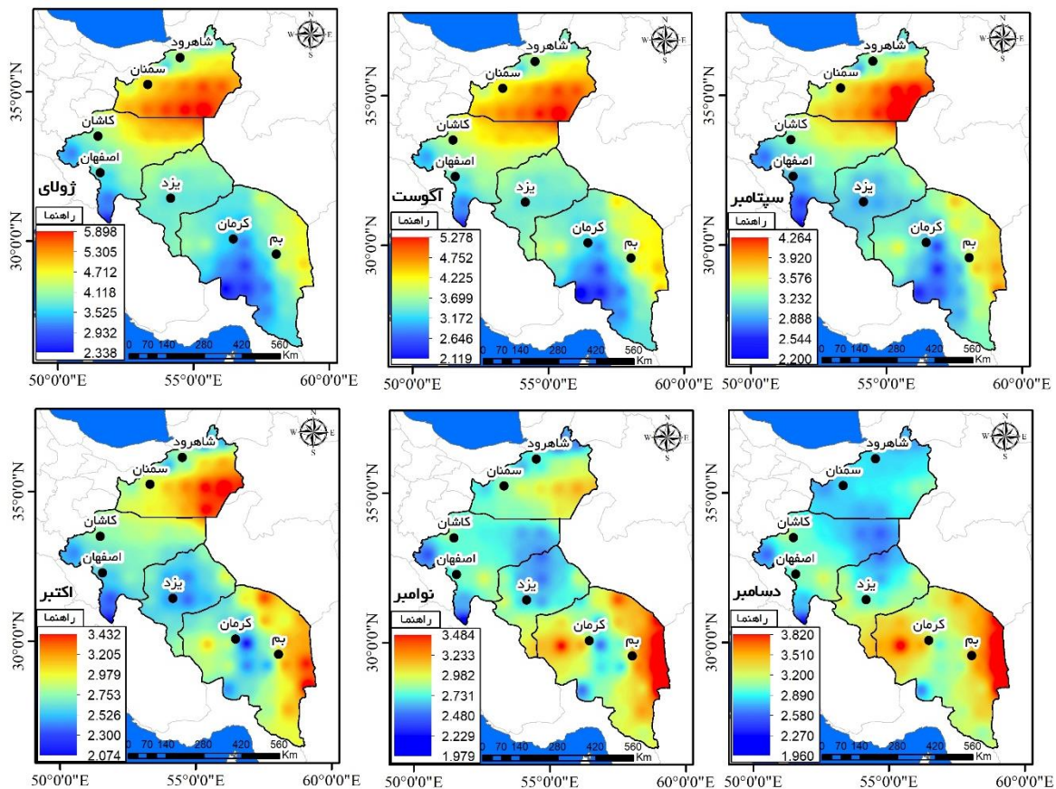
شکل ۴. پراکنش مکانی باد (m/s) در ایران مرکزی براساس پایگاه داده ECMWF نسخه ERA-Interim
