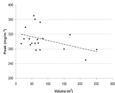
شکل ۴ - همبستگی حداکثر تراکم MMA با حجم لا براتوارها
