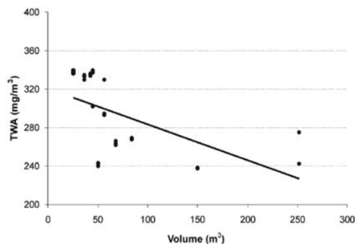
شکل ۳- همبستگی میانگین وزنی MMA با حجم لابراتوارها
