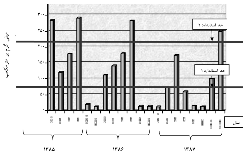
نمودار ۱: غلظت مقایسه ای ذرات معلق خروجی از دودکش های صنایع فرآورده های نسوز سال های ۸۷-۸۵
