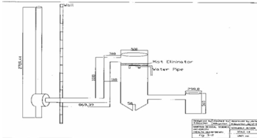
شکل ۱: مشخصه های فنی سیستم پایلوت
