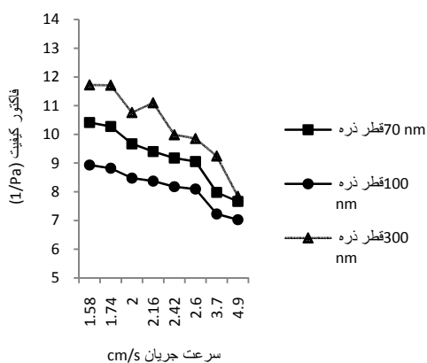
شکل ۷- فاکتور کیفیت (QF) صافی اولپا برای ذرات در گستره ۷۰، ۱۰۰ و ۳۰۰ نانومتر در سرعت جریان ۱.۵۸ تا cm \cdot s^{-1} 5
