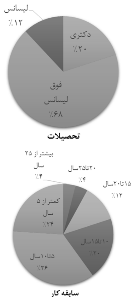
شکل ۳- آمارمیزان تحصیلات و تجربه کاری پاسخ‌دهندگان پرسشنامه
