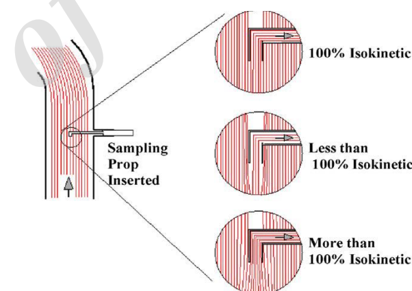
شکل ۲- نمونه‌برداری ایزوکینتیک و غیر ایزوکینتیک
