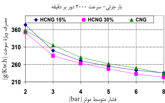
شکل ۱۰ بازده حرارتی در وضعیت بار جزئی برای فشارهای مؤثر متوسط (BMEP) مختلف در سرعت ۲۰۰۰ دور در دقیقه
