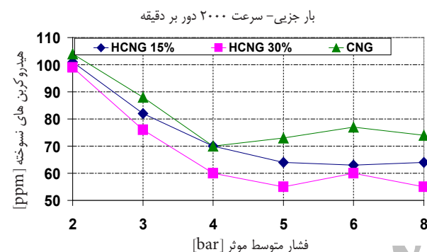
شکل ۱۳ تغییرات آلایندة هیدروکربن‌های نسوخته نسبت به تغییر فشار مؤثر
