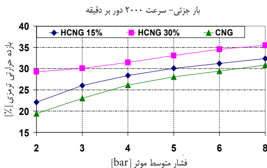
شکل ۹ بازده حرارتی در وضعیت بار جزئی برای فشارهای مؤثر متوسط (BMEP) مختلف در سرعت ۲۰۰۰ دور در دقیقه
