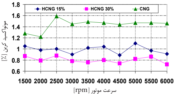
شکل ۵ تغییرات آلایندة مونوکسید کربن بر حسب دور برای سوخت‌های استفاده شده
