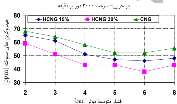
شکل ۱۴ تغییرات آلایندة هیدروکربن‌های نسوخته نسبت به تغییر فشار مؤثر متوسط واقعی در سرعت ۳۰۰۰ دور بر دقیقه برای سوخت‌های مختلف
