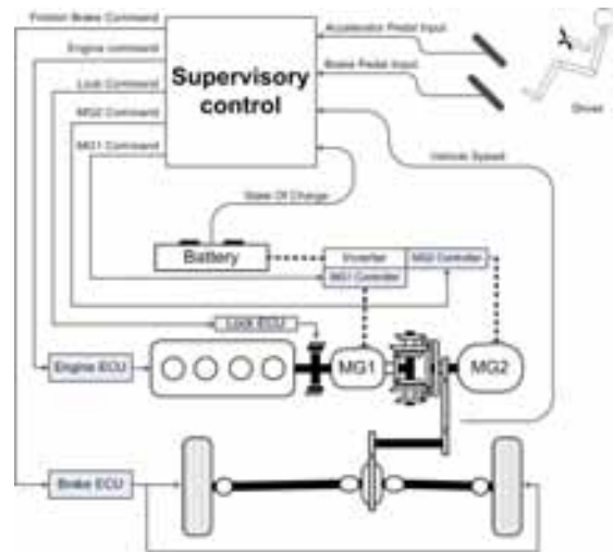
شکل ۴ عملکرد و پایش سامانه دورگه جدید
