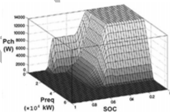
شکل ۱۰ توابع ذخیره انباره برای حد ذخیره‌ها و توان‌های درخواستی مختلف
