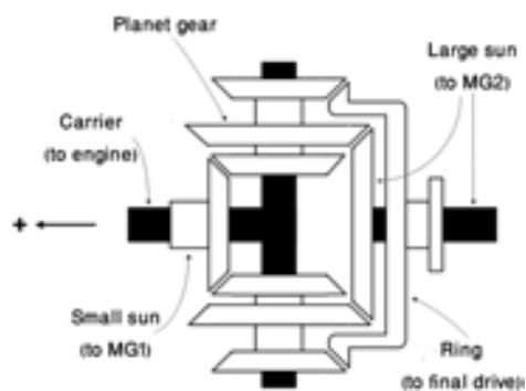
شکل ۲ مجموعه تقسیم کننده توان جدید
