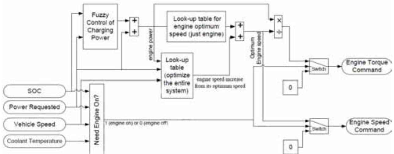
شکل ۶ ساختار پایشگر
