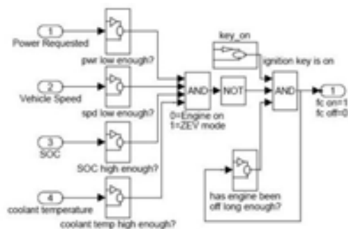
شکل ۷ بلوک دیاگرام خاموش و روشن شدن موتور احتراقی
