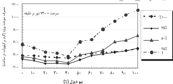
شکل ۵ تأثیر سوخت بیودیزل بر مصرف ویژه سوخت ترمزی در بارهای مختلف موتور و سرعت ثابت ۷۳۰ دور بر دقیقه
