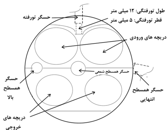
شکل ۱۱ مکان قرارگیری حسگرها در استوانه چهارم [۷]
