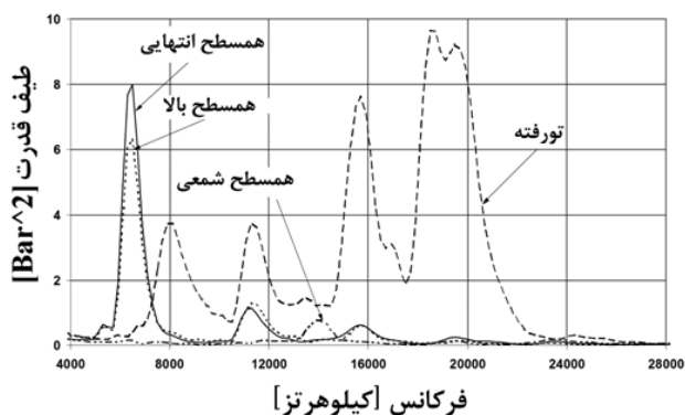
شکل ۱۳ مقایسه منحنی‌های طیف قدرت برای چهار حسگر به طور همزمان [۷]
