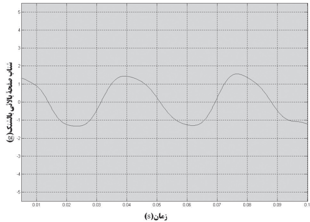
شکل ۲۰ نمودار شتاب صفحه بالایی بالشتک در تحلیل عنصر محدود آزمون‌های حالت ایستایی در نرم افزار آباکوس
