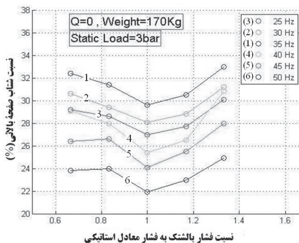
شکل ۱۵ نمودار معرف درصد کاهش شتاب صفحه بالائی بر حسب نسبت فشار با جرم ۱۷۰ کیلوگرمی صفحه بالائی
