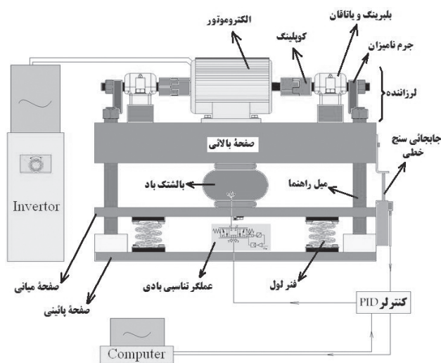
شکل ۱۰ چیدمان طراحی شده برای آزمایش
