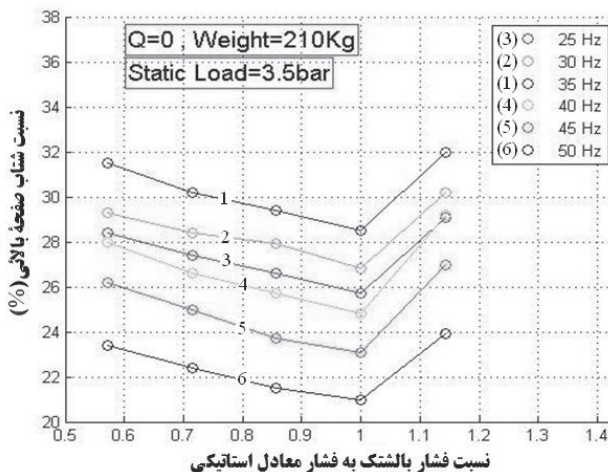
شکل ۱۷ نمودار معرف درصد کاهش شتاب صفحه بالائی بر حسب نسبت فشار با جرم ۲۱۰ کیلوگرمی صفحه بالائی
