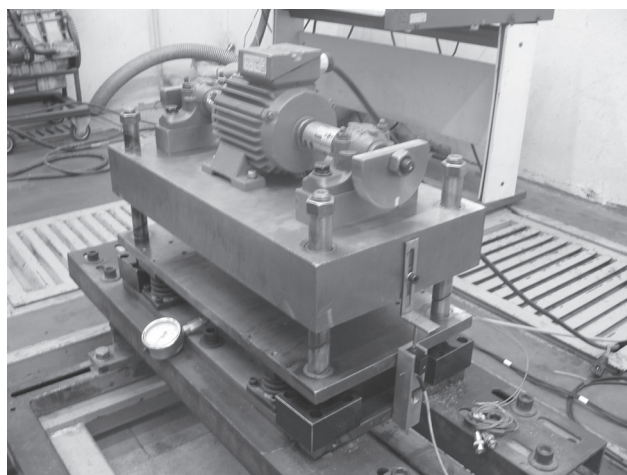
شکل ۱۱ چیدمان ساخته شده برای آزمایش
