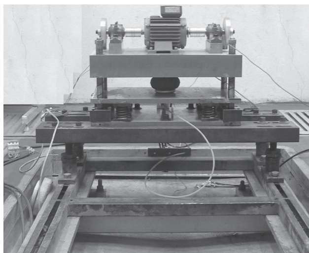
شکل ۱۲ موقعیت قرار گیری بالشتک و دیگر اجزای چیدمان آزمایش
