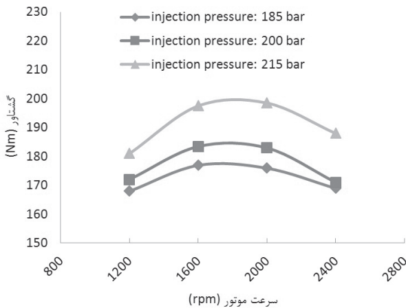
شکل ۶ گشتاور برحسب سرعت موتور برای سوخت B100 به ازای مقادیر مختلف فشار پاشش
