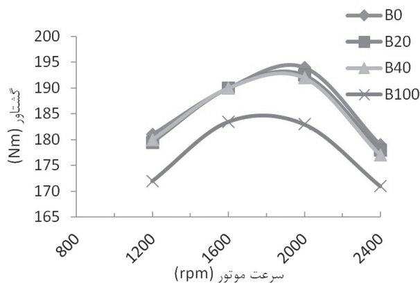
شکل ۴ گشتاور برحسب سرعت موتور برای مخلوط‌های مختلف سوخت‌های دیزل و بیودیزل
