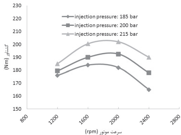
شکل ۴ گشتاور برحسب سرعت موتور برای سوخت B20 به ازای مقادیر مختلف فشار پاشش
