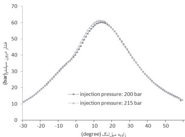
شکل ۱۳ فشار درون استوانه برحسب زاویه میل‌لنگ برای سوخت B۲۰ به ازای دو مقدار مختلف فشار پاشش
