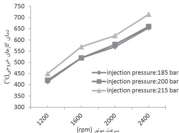
شکل ۱۲ دمای گازهای خروجی از مجرای دود برحسب سرعت موتور برای سوخت B۱۰۰ به ازای مقادیر مختلف فشار پاشش
