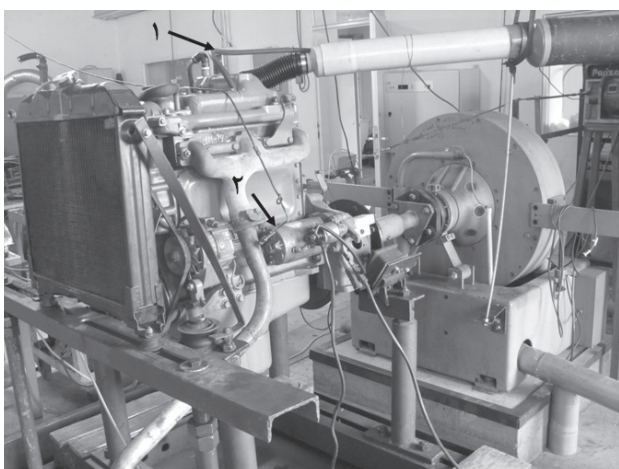
شکل ۱ بستر آزمون موتور مجهز به لگام‌ترمز جریان گردابی، (۱) سیم انتقال علامت فشار درون استوانه، (۲) ترموکوپل
