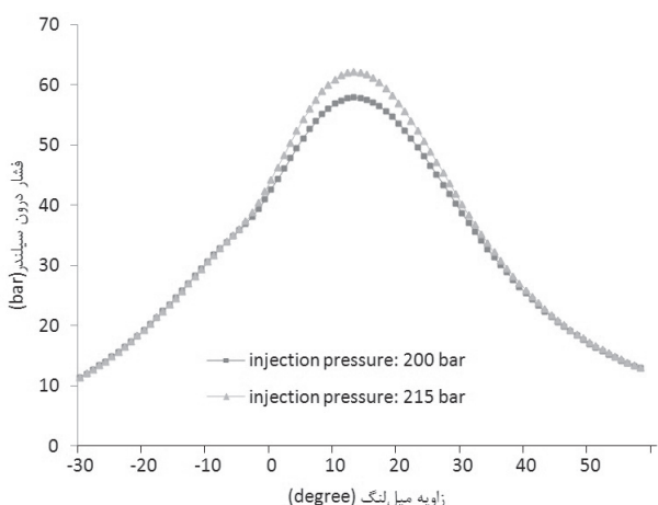
شکل ۱۵ فشار درون استوانه برحسب زاویه میل‌لنگ برای سوخت B۱۰۰ به ازای دو مقدار مختلف فشار پاشش
