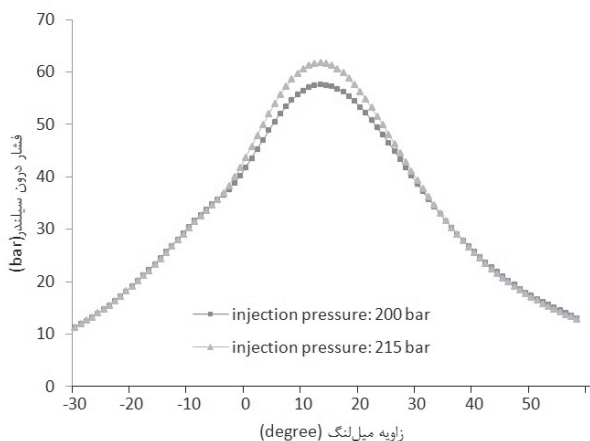
شکل ۱۴ فشار درون استوانه برحسب زاویه میل‌لنگ برای سوخت B۴۰ به ازای دو مقدار مختلف فشار پاشش
