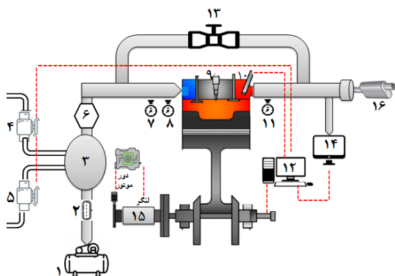
شکل ۴: شماتیکی از تجهیزات آزمون و محل قرار گیری حسگرها
