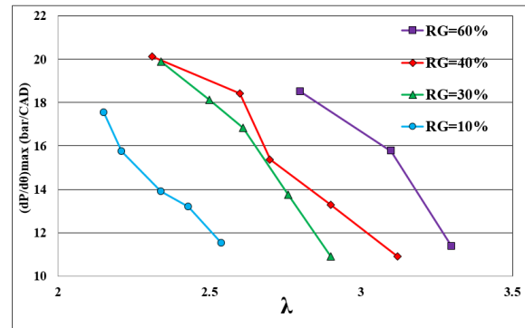
شکل ۱۰: تأثیر نسبت گاز تبدیل بر حداکثر نرخ افزایش فشار داخل محفظه در نتایج تجربی
