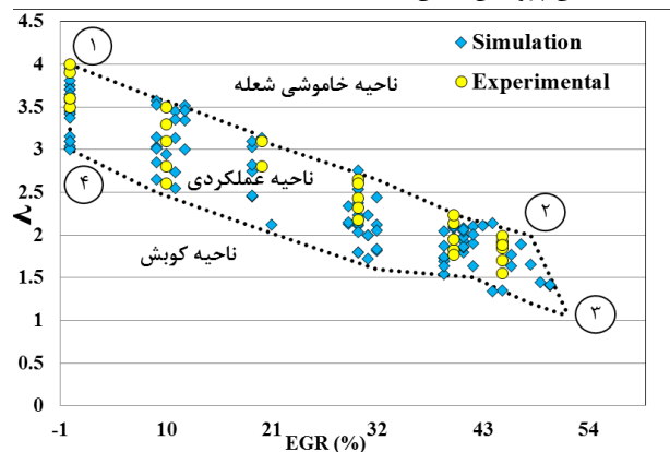
شکل ۵: بازه عملکردی \lambda -EGR برای احتراق HCCI گاز طبیعی با دمای اولیه و نسبت تراکم
