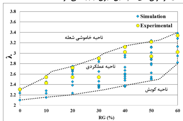
شکل ۸: تأثیر گاز تبدیل بر گسترش بازه عملکردی موتور با احتراق HCCI گاز طبیعی
