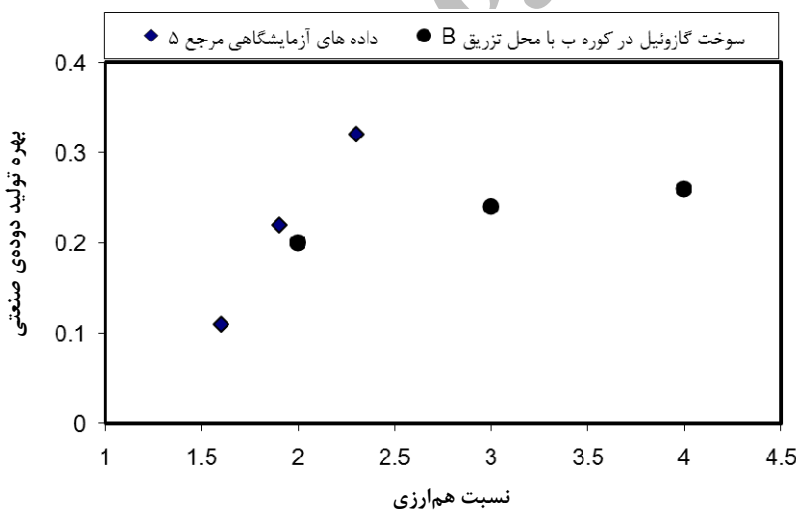
شکل ۷- مقایسه‌ی نتایج سوخت گازوئیل با نتایج مرجع [۵]
