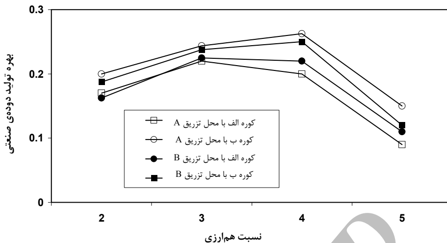
شکل ۶- بهره تولید سوخت گازوئیل در شرایط مختلف کوره
