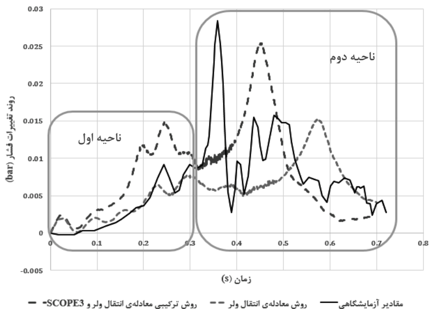
شکل ۴- مقایسه نمودار نتایج عددی روش احتراقی ترکیبی با معادله انتقال ولر در محاسبه تغییرات فشار حاصل از انفجار مخلوط استوکیومتریک پروپان/هوا در مقیاس بزرگ و آغازش از وسط محفظه
