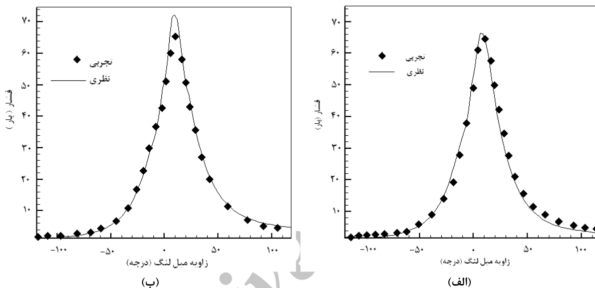
شکل ۱- مقایسه تغییرات فشار داخل محفظه احتراق بر حسب زاویه میل لنگ برای حالت نظری و تجربی برای (الف) دور گشتاور بیشینه (۱۴۰۰ دور بر دقیقه) و (ب) برای دور ۱۲۰۰ دور بر دقیقه
