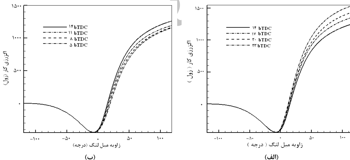
شکل ۵- تغییرات اگزرژی کار مبادله شده با تغییر زمان پاشش، الف: پاشش نسبت به حالت پایه زودتر شروع شده است. ب: پاشش نسبت به حالت پایه به تعویق انداخته شده است.
