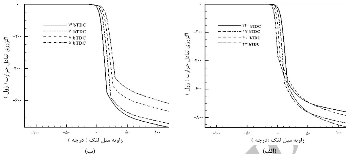
شکل ۴- تغییرات اگزرژی حرارت منتقل شده با تغییر زمان پاشش برای دور گشتاور بیشینه (۱۴۰۰ دور بر دقیقه)، الف: پاشش نسبت به حالت پایه زودتر شروع شده است. ب: پاشش نسبت به حالت پایه به تعویق انداخته شده است.
