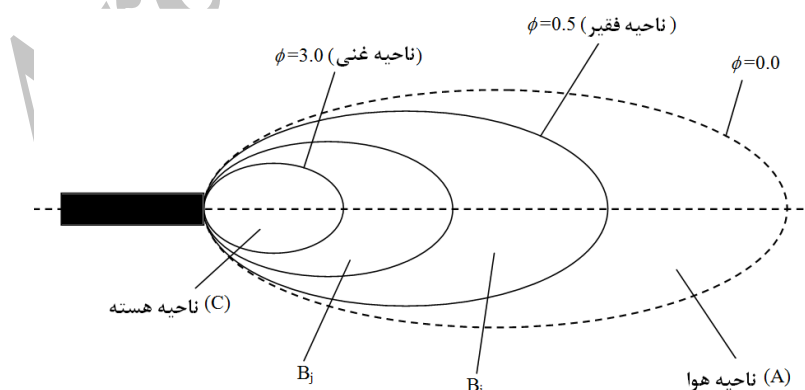
شکل ۱- جزئیات مدل احتراقی چندمنطقه‌ای کامینز (Cummins)
