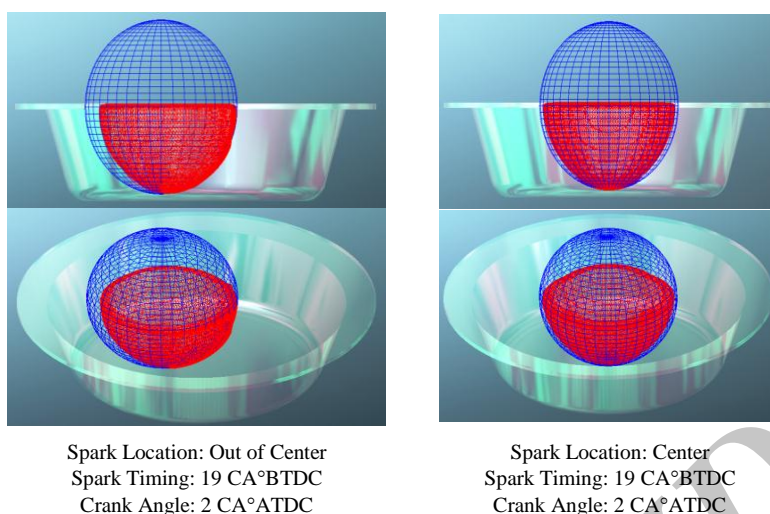
Figure 6- Comparison of real flame surface and assumed spherical flame growth in both center and off-center spark plug position شکل ۶- مقایسه سطح شعله واقعی نسبت به شعله با فرض رشد کروی برای هر دو حالت شمع جرقه در مرکز و خارج از مرکز
