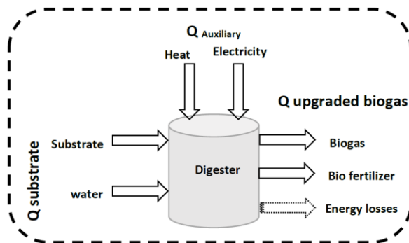
Figure 7- A schematic view of the energy balance & boundary of the system considered for the biogas reactor شکل ۷- نمای طرحواره مرز سیستم و موازنه انرژی در نظر گرفته شده برای راکتور بیوگاز
