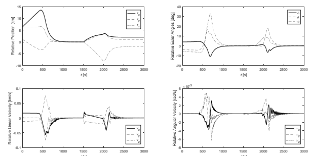
شکل ۹- مسیرهای حالت کنترل‌شده با PSCP-SPCA
