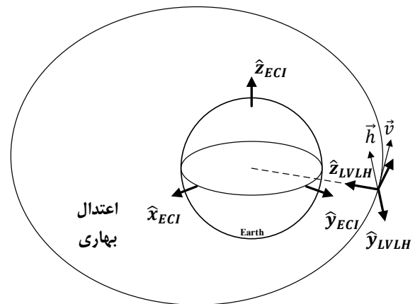
شکل ۱- دستگاه‌های مختصات ECI و LVLH ( \vec{h} و \vec{v} به ترتیب عبارتند از بردارهای سرعت خطی و ممتوم زاویه‌ای مداری)
