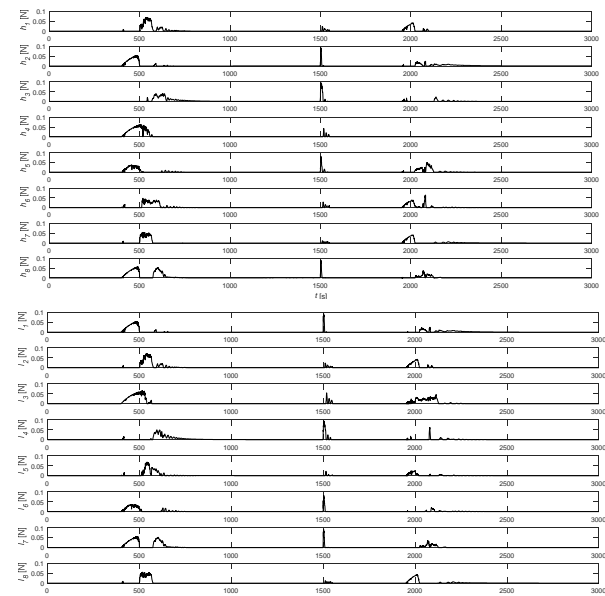
شکل ۱۶ - رانش تولید شده توسط هر رانشگر در PSPCCA
