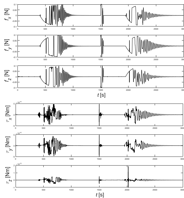
شکل ۱۲- نیرو و گشتاور برآیند تولید شده توسط PSCP-SPCA
