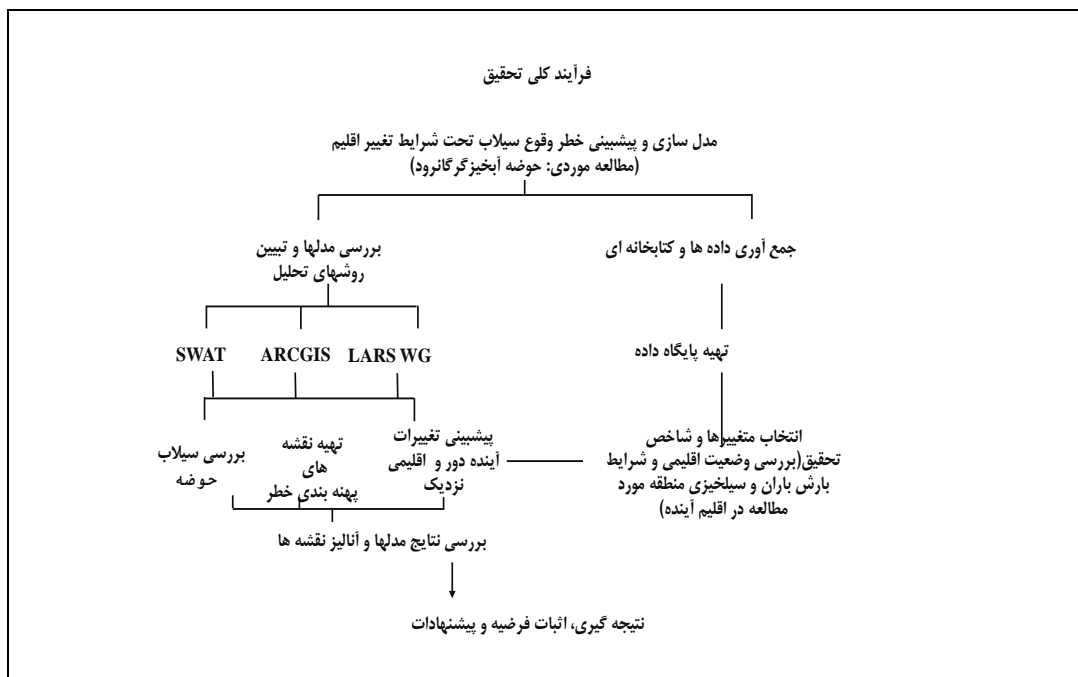
شکل ۳. فرایند تحقیق پهنه بندی منطقه ای سیلاب با استفاده از روش سلسله مراتبی و مدل هیدرولوژیکی SWAT منبع: (ترسیم نگارندگان ۱۴۰۱)
