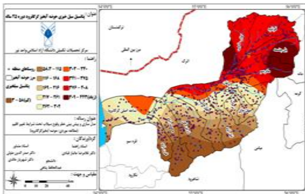
شکل ۵. پهنه بندی خطر سیلاب آینده با استفاده از خروجی روش SWAT دوره ۲۵ ساله منبع: (ترسیم نگارندگان، ۱۴۰۱)
