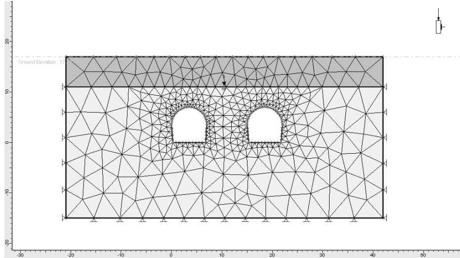
شکل (۸): مدل سازی تونل های قطار شهری به منظور تحلیل عددی
