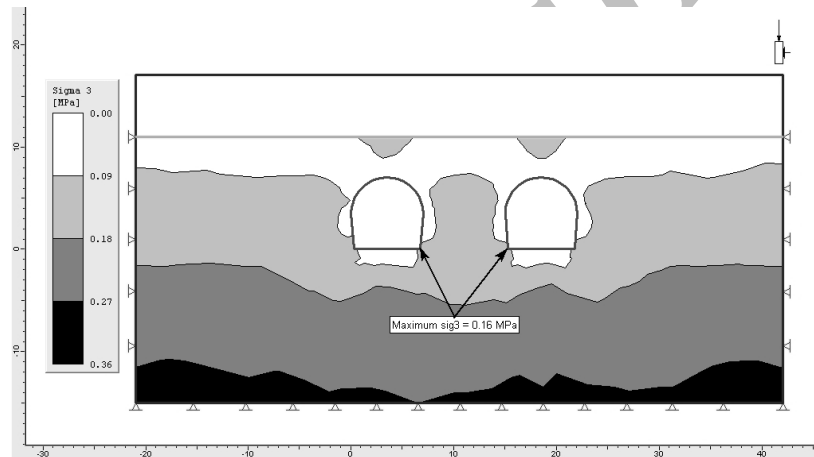
شکل (۱۱): تنش‌های القایی حداقل در تونل‌های قطار شهری اصفهان در حدفاصل ایستگاه آزادی-دانشگاه
