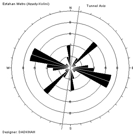
شکل ۲: نمودار رزدياگرام ناپيوستگي ها در توده سنگ های حدفاصل ایستگاه آزادی-دانشگاه
