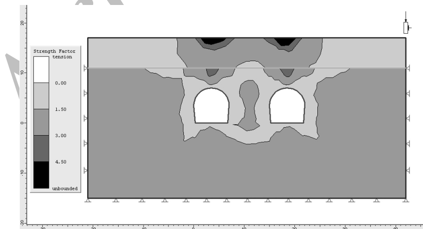
شکل (۱۲): فاکتور مقاومت در اطراف تونل‌های قطار شهری اصفهان در حدفاصل ایستگاه آزادی-دانشگاه
