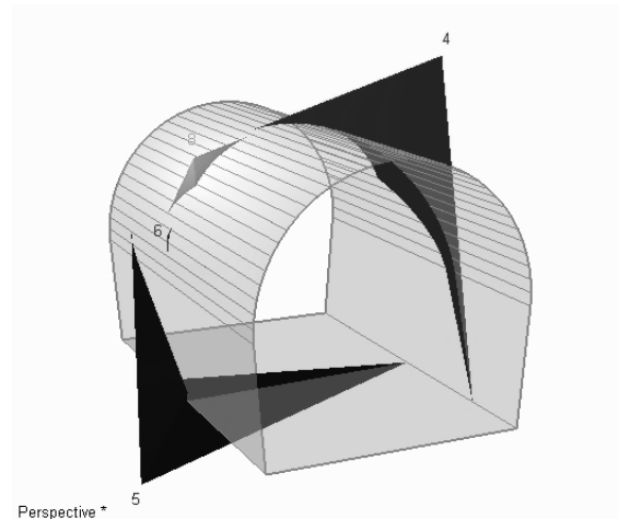
شکل (۷): گوه‌های شناسایی شده در امتداد تونل در حد فاصل ایستگاه آزادی-دانشگاه
