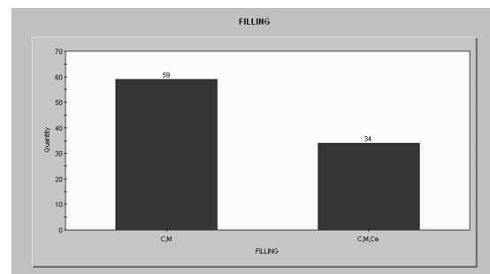
شکل ۵: آنالیز آماری پرشدگی ناپیوستگی‌ها در توده‌سنگ‌های حدفاصل ایستگاه آزادی-دانشگاه (Ca=Calcite M=Silt C=Clay)
