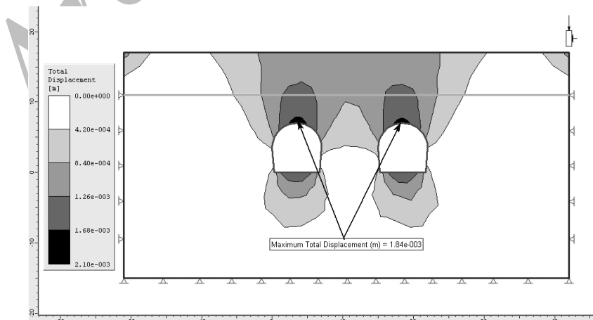
شکل (۱۴): جابجایی حداکثر در اطراف تونل های قطار شهری اصفهان در حدفاصل ایستگاه آزادی-دانشگاه
