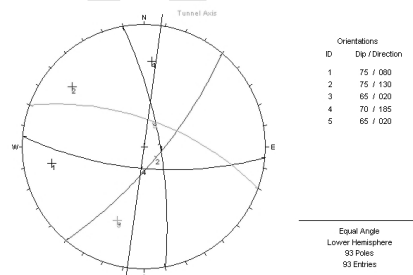
شکل ۱: تصویر استریوگرافی ناپيوستگي های موجود در توده سنگ های حدفاصل ایستگاه آزادی-دانشگاه
