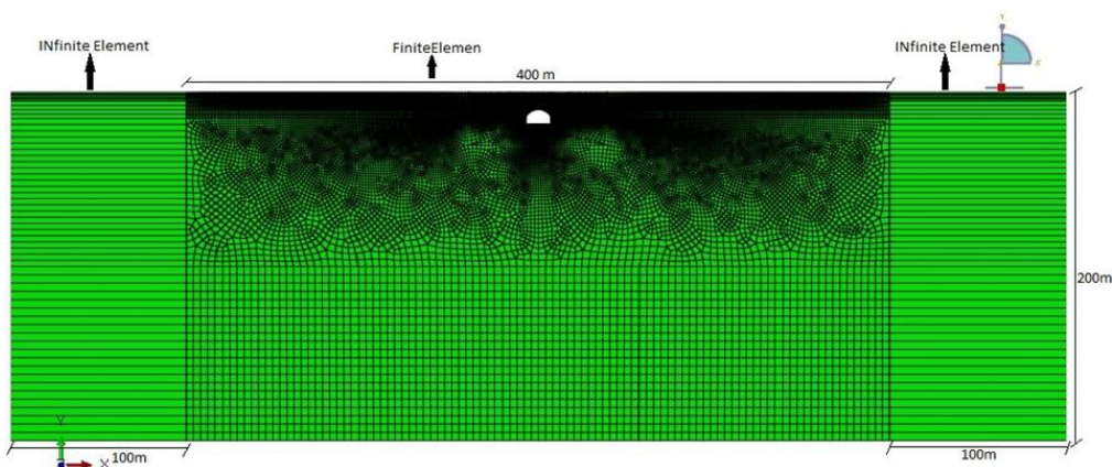
شکل 3. پیکره و ابعاد مدل دوبعدی مورد استفاده در نرم‌افزار آباکوس به منظور تحلیل عددی اثر حفره بر پاسخ لرزه‌ای زمین
