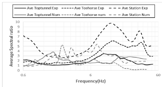
شکل 6. مقایسه نتایج به روش عددی و تجربی: سمت راست: مقایسه نسبت‌های طیفی میانگین با افزایش ابعاد در مطالعات عددی و تجربی و مشاهده روند افزایشی قله‌ها با بزرگ‌تر شدن ابعاد، سمت چپ: میانگین‌گیری مجدد از نسبت‌های طیفی میانگین در دو روش عددی و تجربی به منظور مشاهده تفاوت‌های میان آن‌ها. ( Exp : نتایج تجربی، Num : نتایج عددی)
