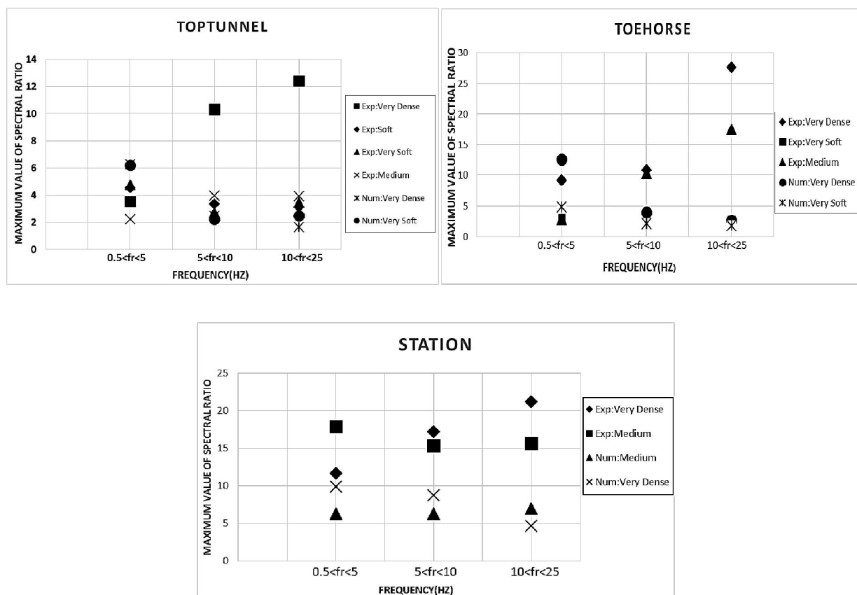
شکل 10. مقادیر حداکثر قله‌های نسبت طیفی در بازه‌های فرکانسی مختلف، دسته‌بندی شده بر اساس خصوصیات ژئوتکنیکی مختلف در سه شکل مقطع فوقانی، نعل اسبی و ایستگاه کامل
