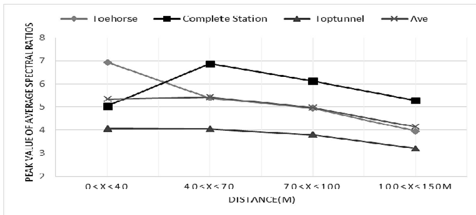
شکل 7. مقادیر حداکثر نسبت‌های طیفی میانگین در بازه فرکانسی بین 0/5 تا 15 هرتز در فواصل مختلف از محور حفره
