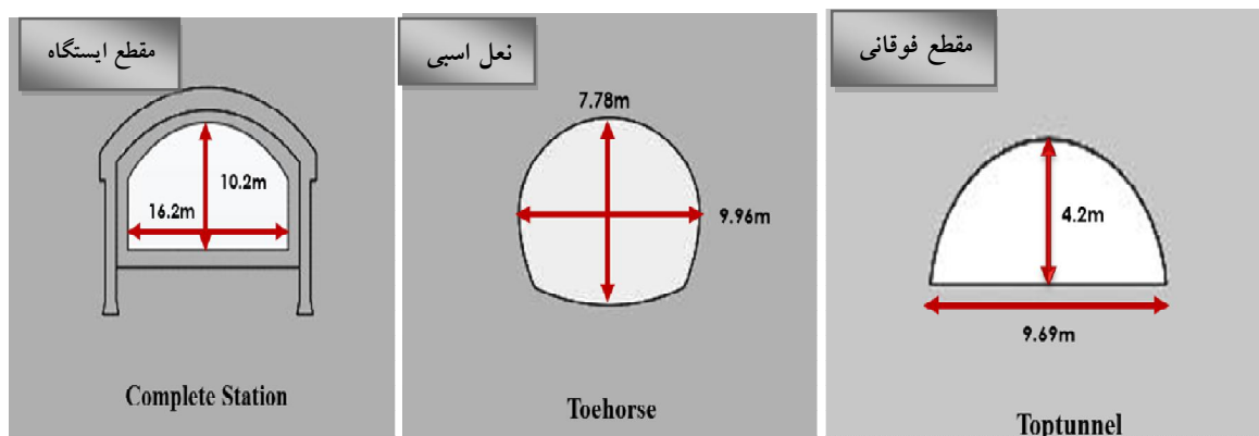
شکل 4. شکل هندسی شماتیک هرکدام از اشکال سه‌گانه تونل مورد اشاره در جدول 1 و ابعاد متناظر با آن‌ها
