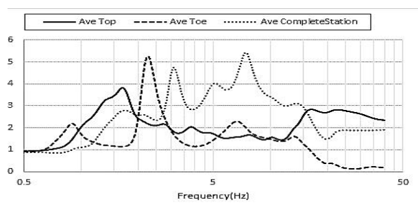
شکل 5. مقایسه نسبت‌های طیفی میانگین سطح به کف در سه شکل مختلف تونل ذکر شده به دست آمده از مدل‌سازی عددی
