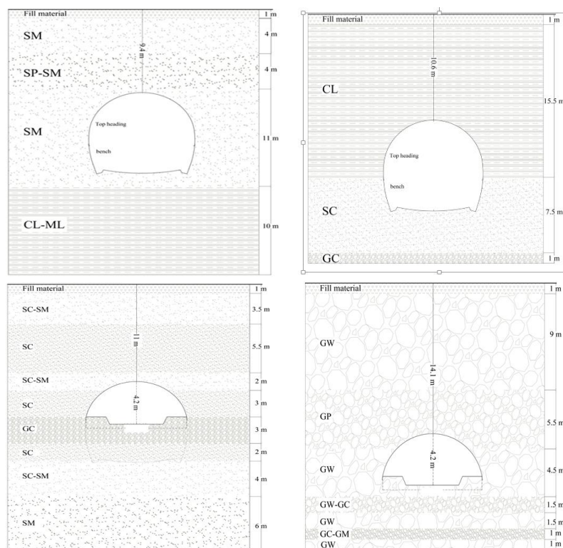
شکل 2. مقایسه پروفیل‌های زیرسطحی مقاطع انتخابی، بالا سمت راست: مقطع ژئوتکنیکی محل N1، بالا سمت چپ: مقطع ژئوتکنیکی محل N2، پایین سمت راست: مقطع ژئوتکنیکی محل N9، پایین سمت چپ: مقطع ژئوتکنیکی محل N4
