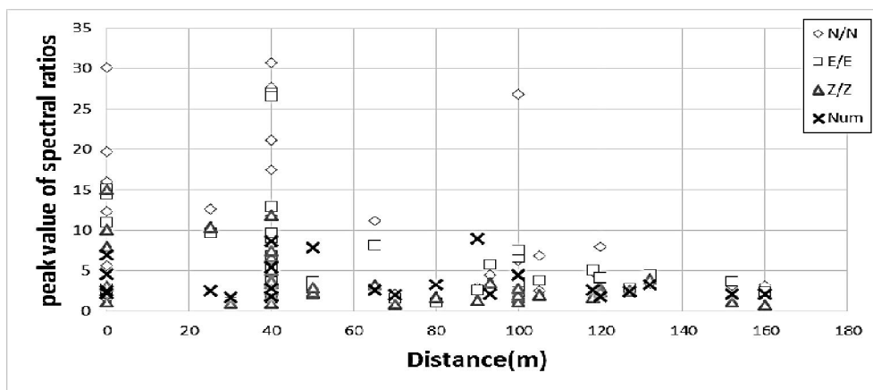
شکل 8. مقایسه مؤلفه‌های حداکثر قله‌های نسبت طیفی در بازه فرکانسی بین 4 تا 20، برای مؤلفه‌های مختلف (N/N، E/E و Z/Z) به دست آمده از اندازه‌گیری تجربی با نتایج به دست آمده از تحلیل عددی. محاسبه در مدل‌سازی عددی تنها برای مؤلفه شمالی - جنوبی صورت گرفته است.
