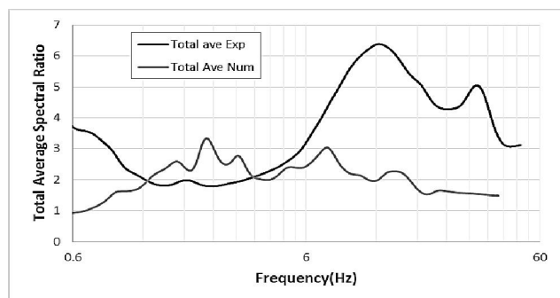
شکل 6. مقایسه نتایج به روش عددی و تجربی: سمت راست: مقایسه نسبت‌های طیفی میانگین با افزایش ابعاد در مطالعات عددی و تجربی و مشاهده روند افزایشی قله‌ها با بزرگ‌تر شدن ابعاد، سمت چپ: میانگین‌گیری مجدد از نسبت‌های طیفی میانگین در دو روش عددی و تجربی به منظور مشاهده تفاوت‌های میان آن‌ها. ( Exp : نتایج تجربی، Num : نتایج عددی)
